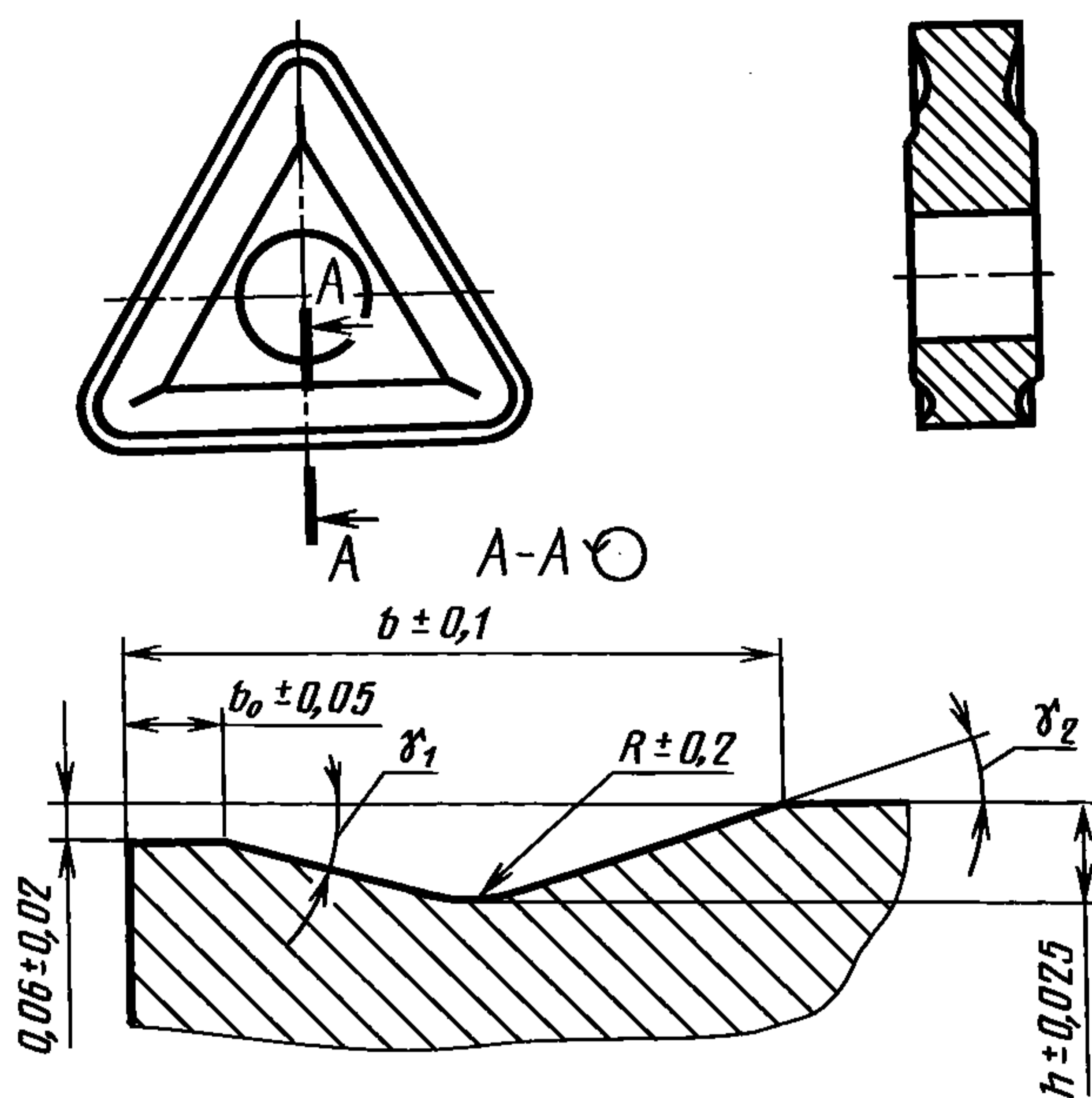
Размеры, мм
