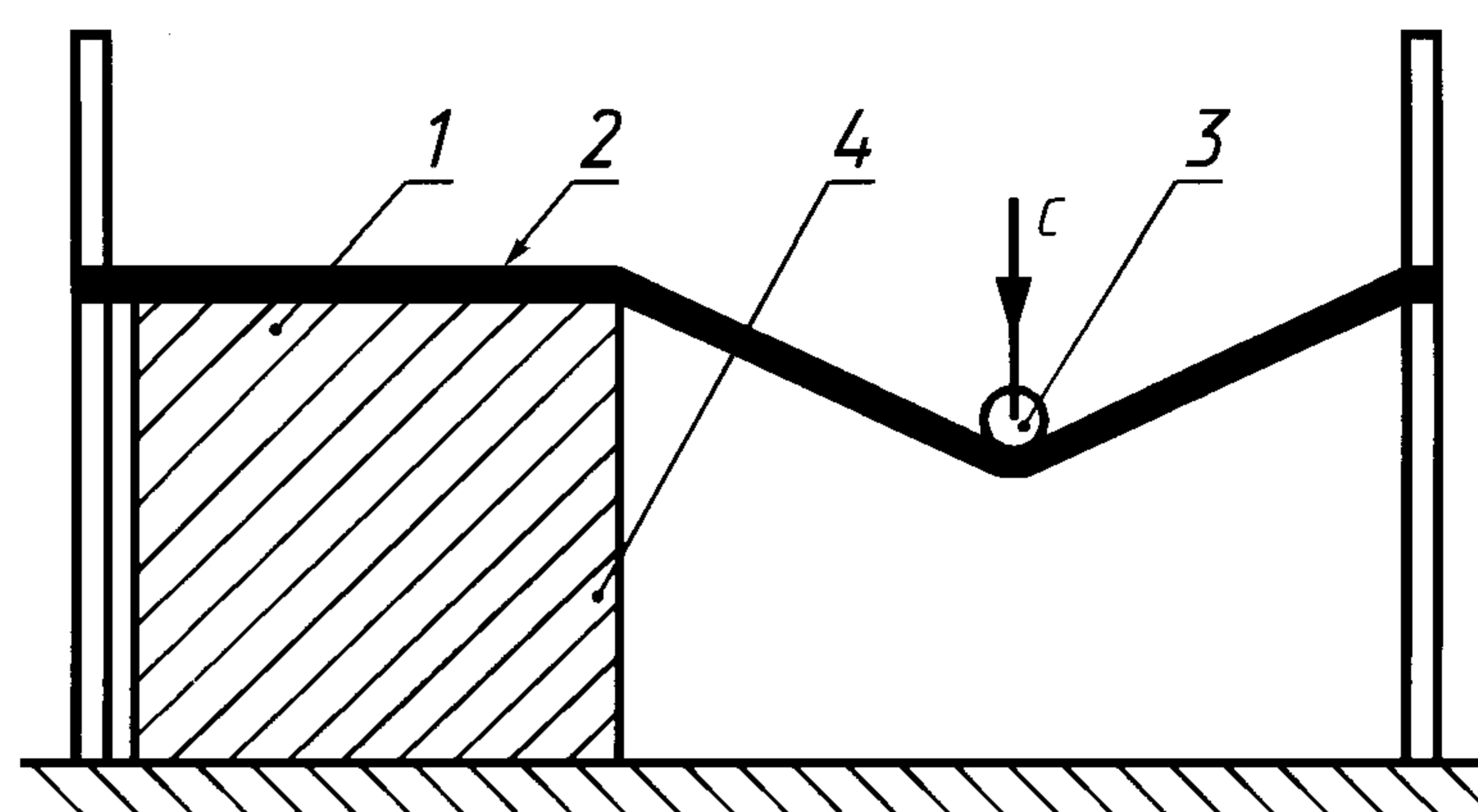
1 — образец; 2 — канат; 3 — ролик; 4 — крышка
