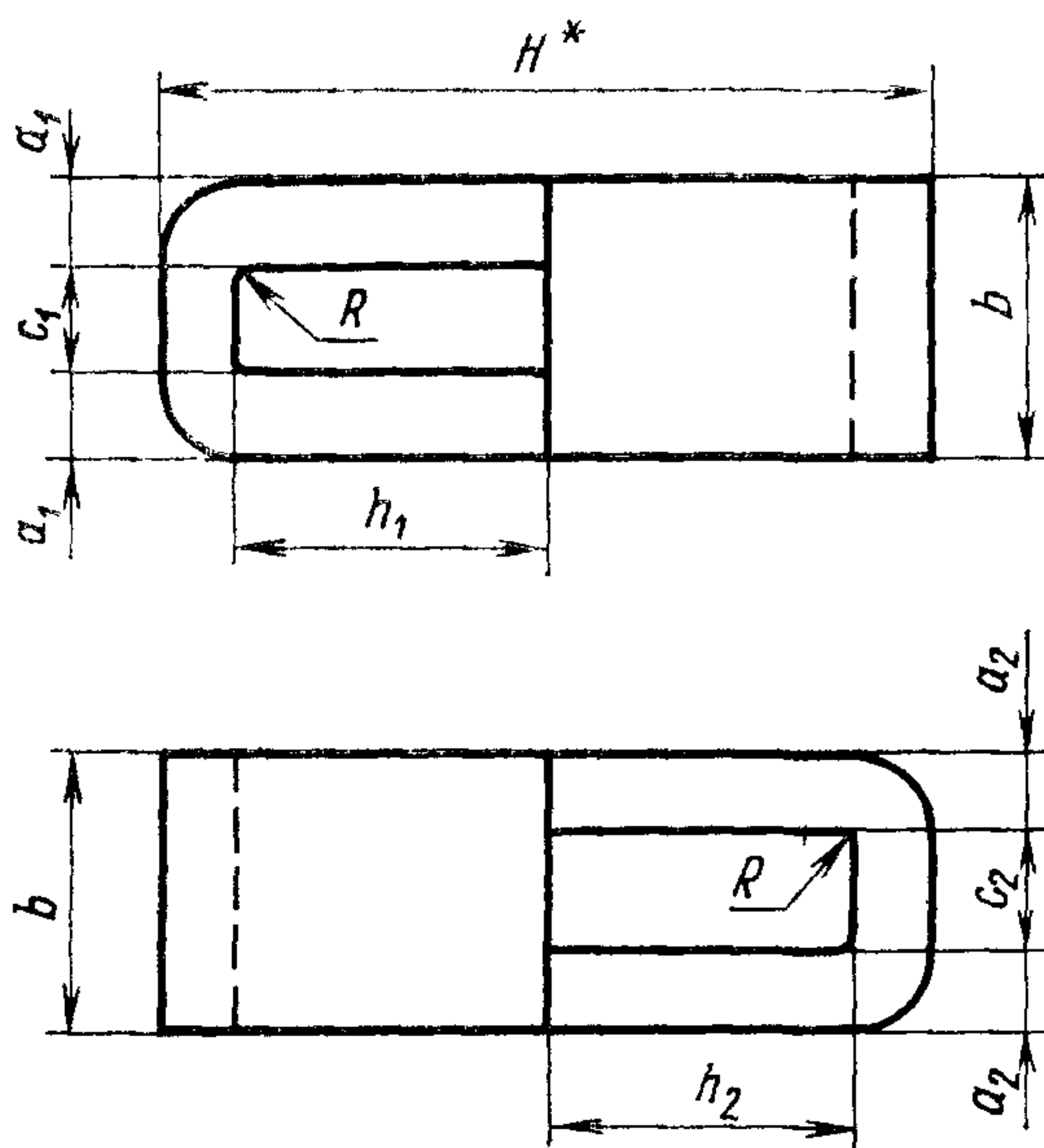
Магнитопроводы ортогональной конструкции
