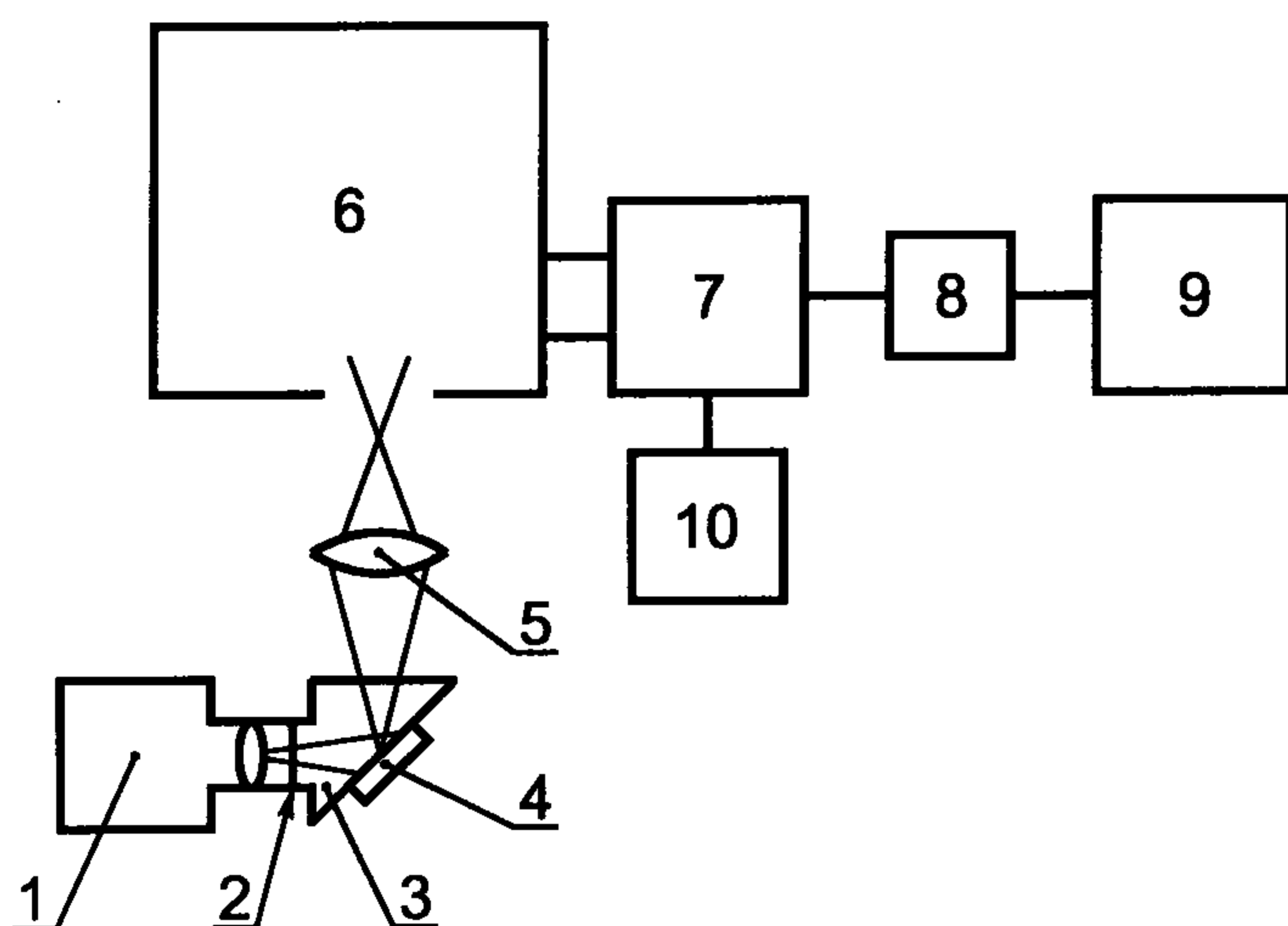
1 — осветитель ОЦ-18 с ртутной лампой ДРШ-250; 2 — свето- фильтр УФС-2; 3 — камера возбуждения; 4 — кювета с кристал- лофосфором; 5 — конденсор; 6 — монохроматор МДР-3; 7 — фотоумножитель ФЭУ-62; 8 — усилитель У5-6; 9 — самописец КСП-4; 10 — высоковольтный выпрямитель ВС-22
