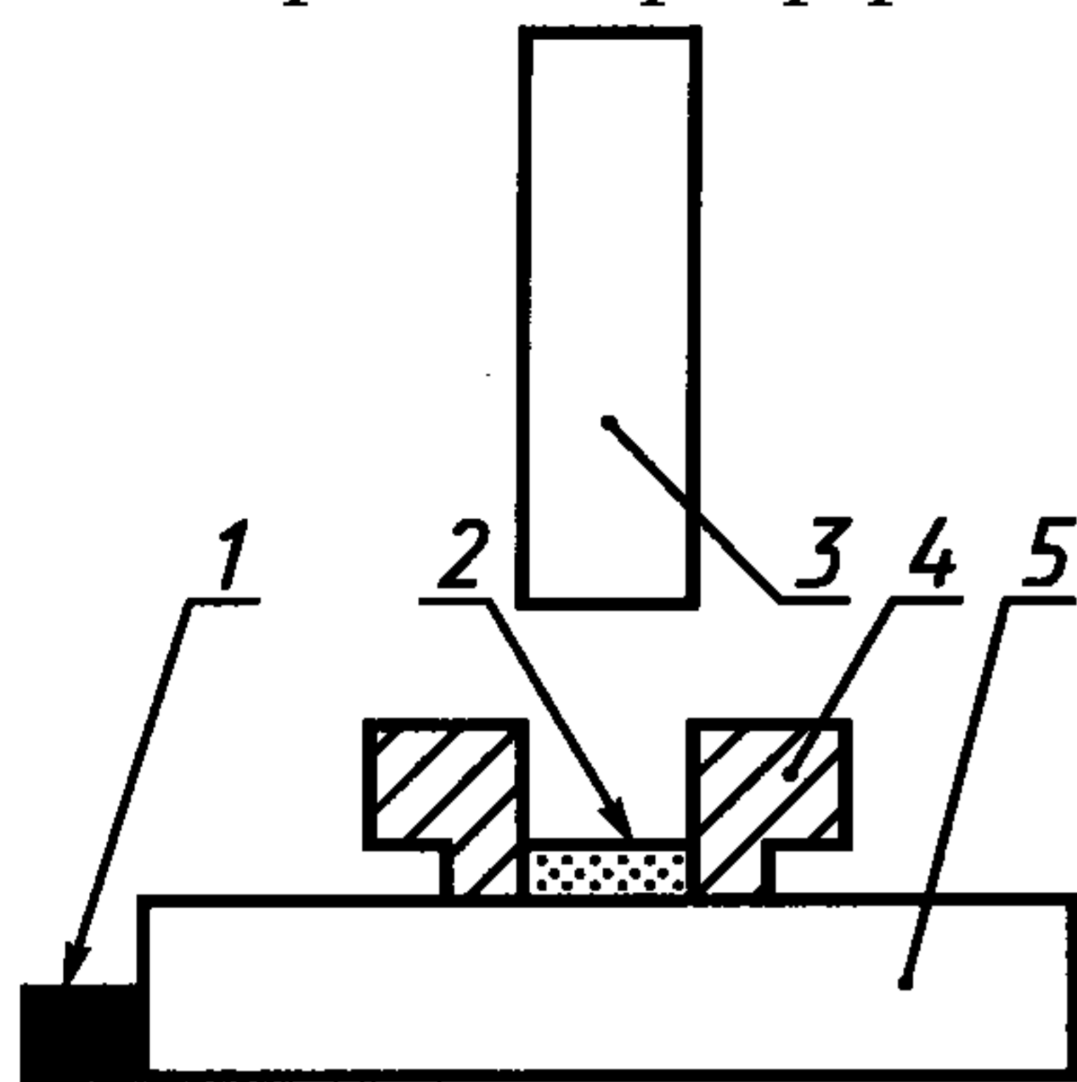
1 — магнит; 2 — образец; 3 — пуансон; 4 — кювета; 5 — подложка
