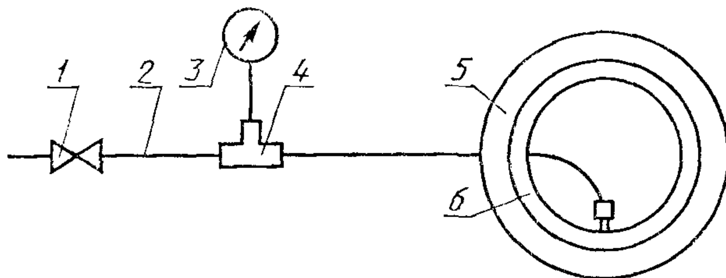
Схема установки для определения потери внутреннего давления в шине
