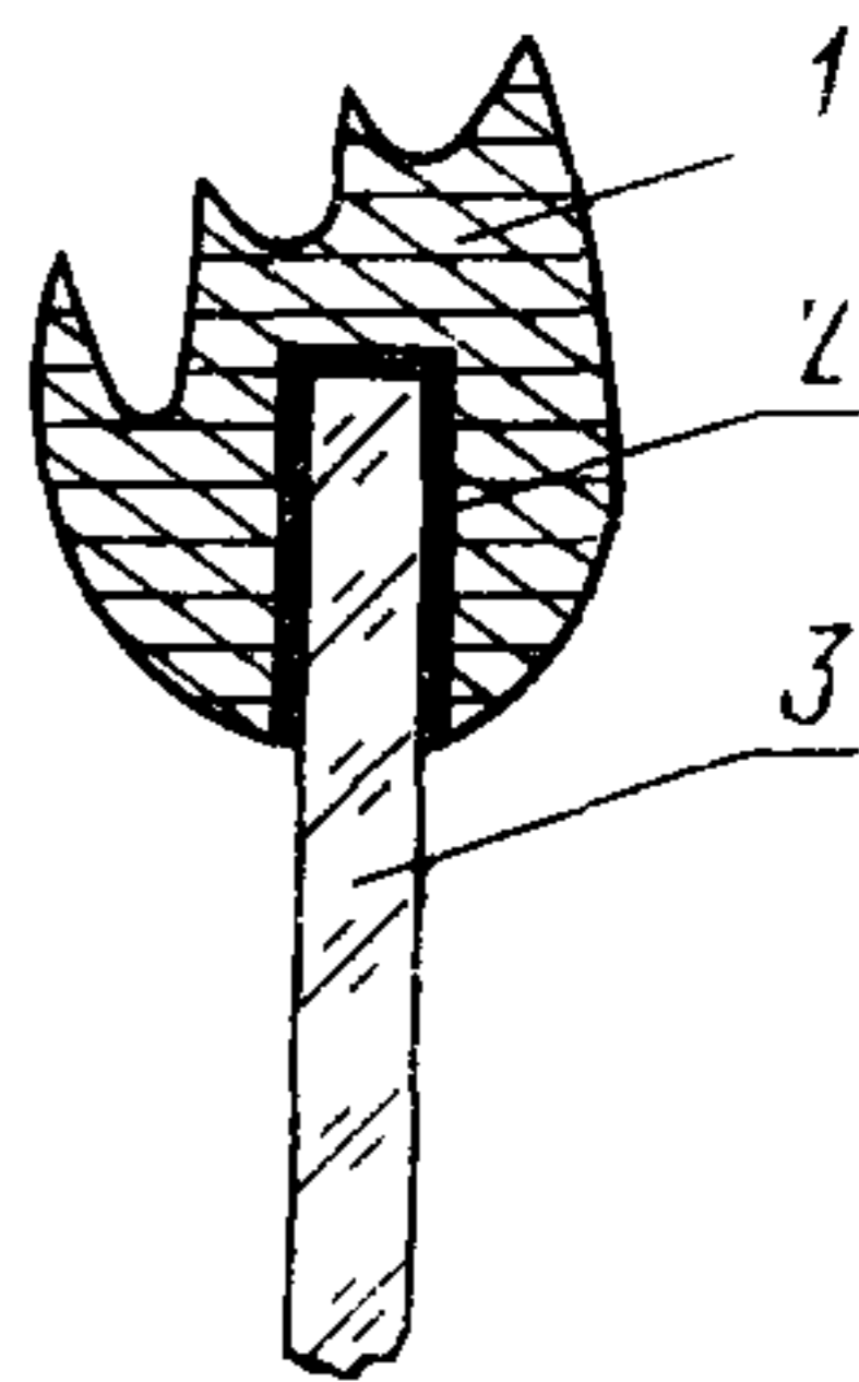
1—резиновый уплотнитель; 2—мастика, 3—стекло
