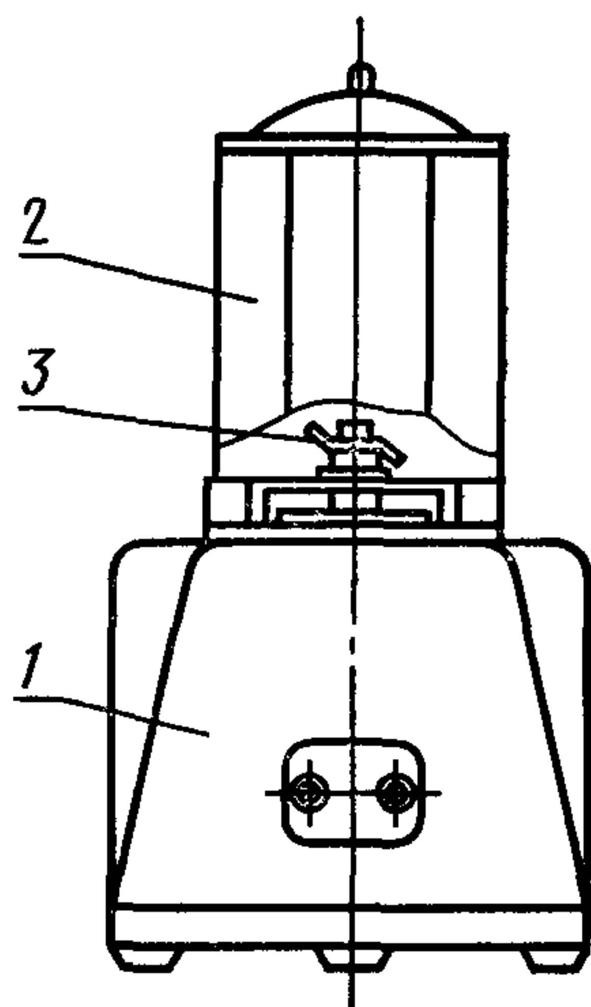
1—привод; 2—мерный стакан; 3—импеллер
