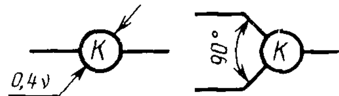
Блок переменного коэффициента
