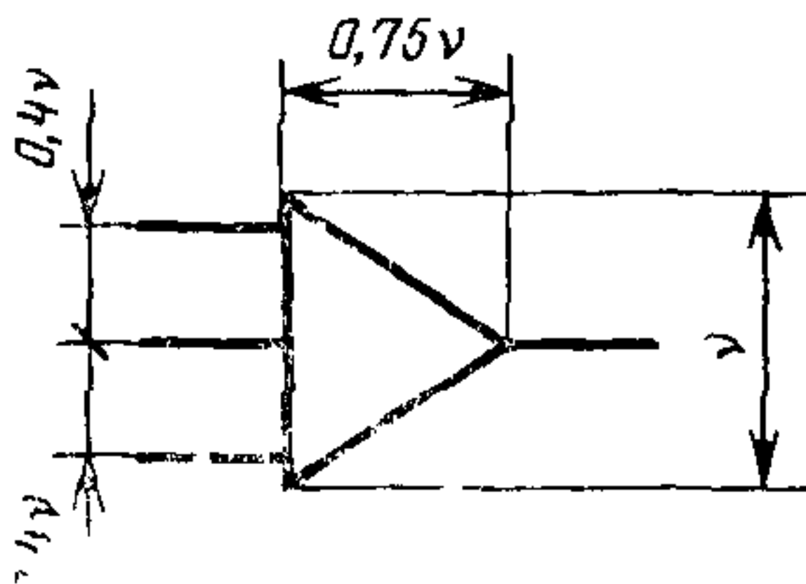
Усилитель суммирующий
