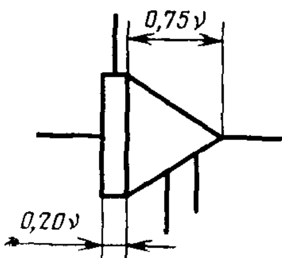
Усилитель дифференцирующий
