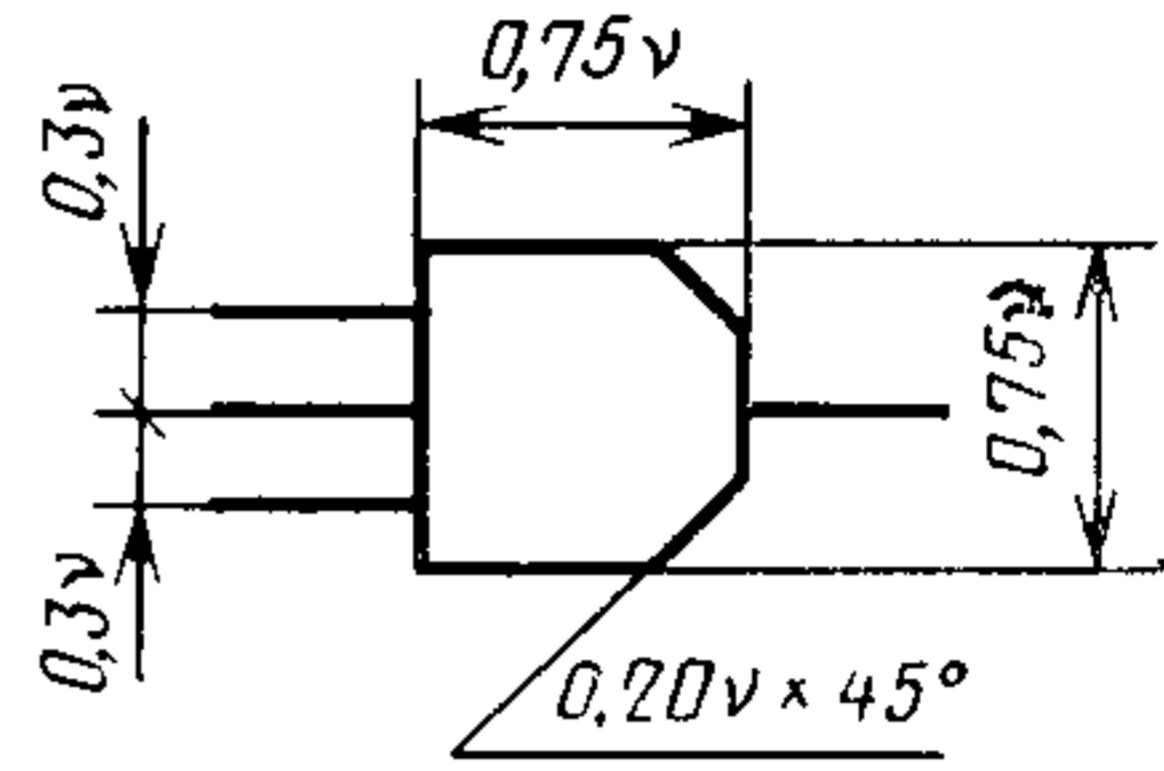
Компаратор
