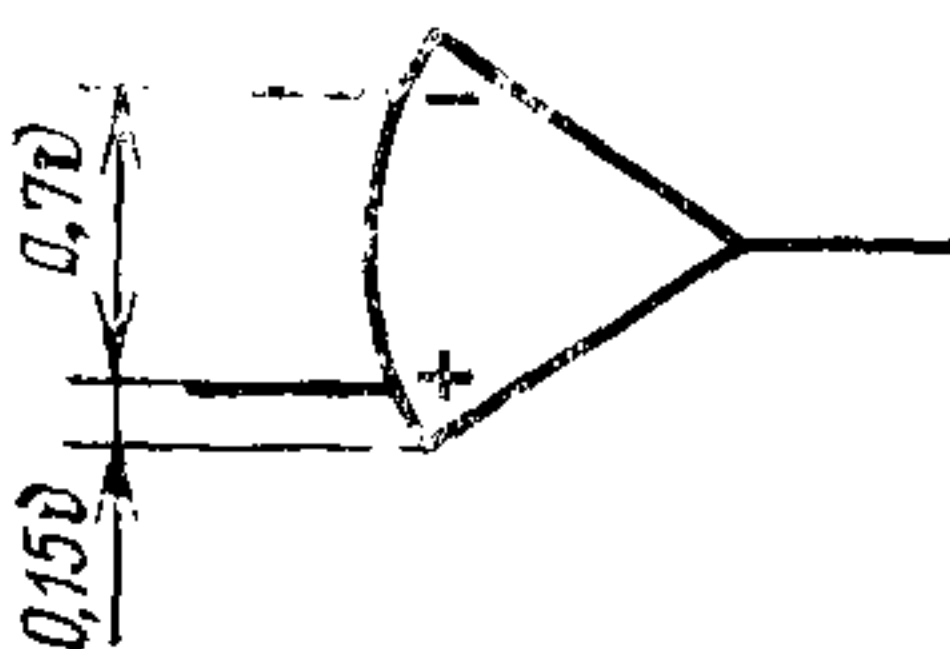
Усилитель операционный с дифференциальным входом
