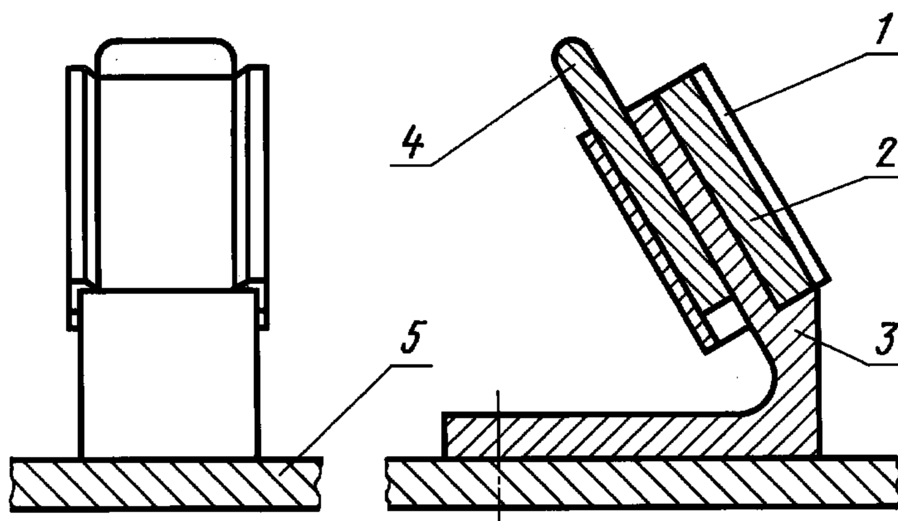
1 — прижимная скоба; 2 — образец; 3 — держатель; 4 — опорное кольцо; 5 — клин
