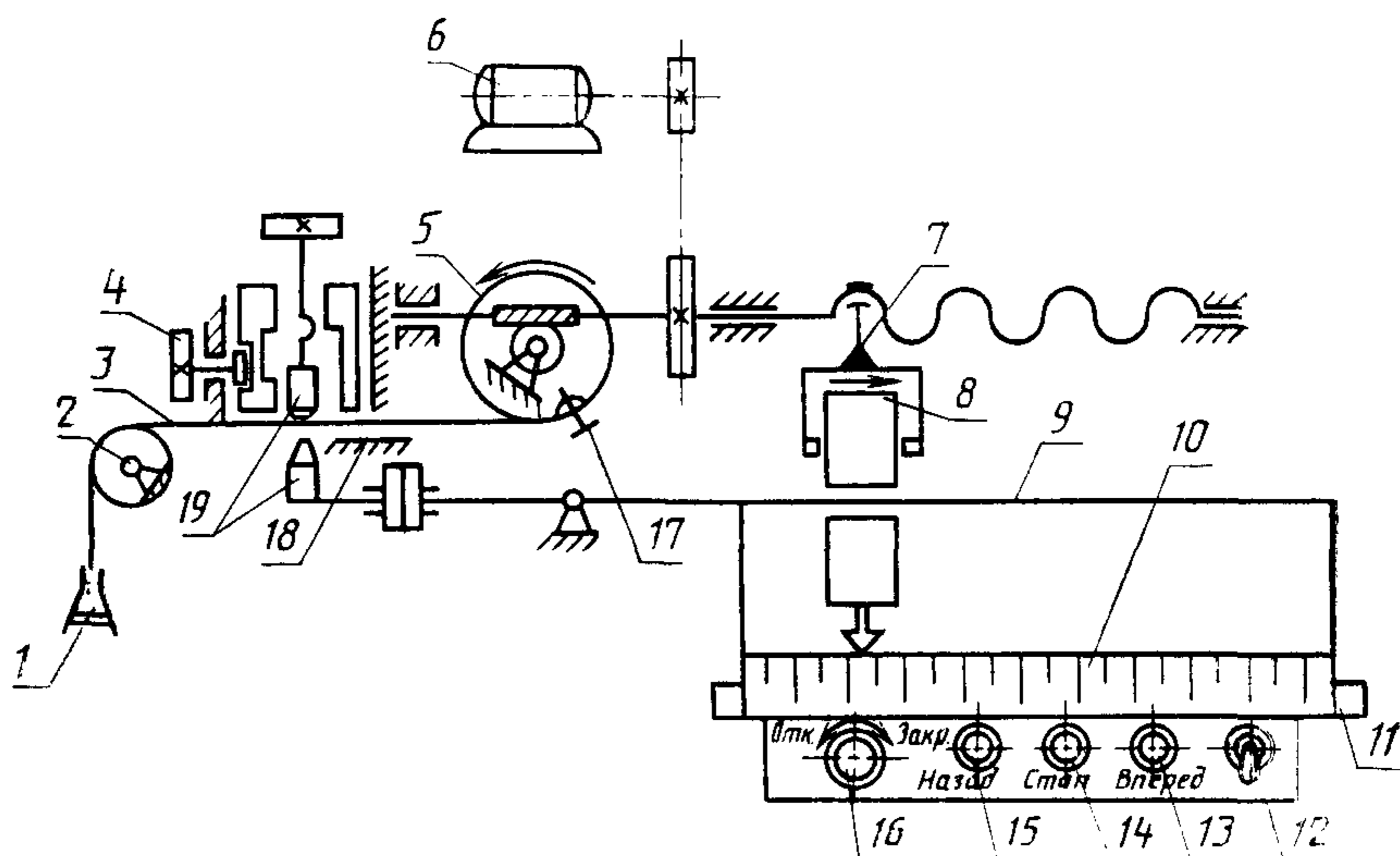
Схема прибора РТ-2М
