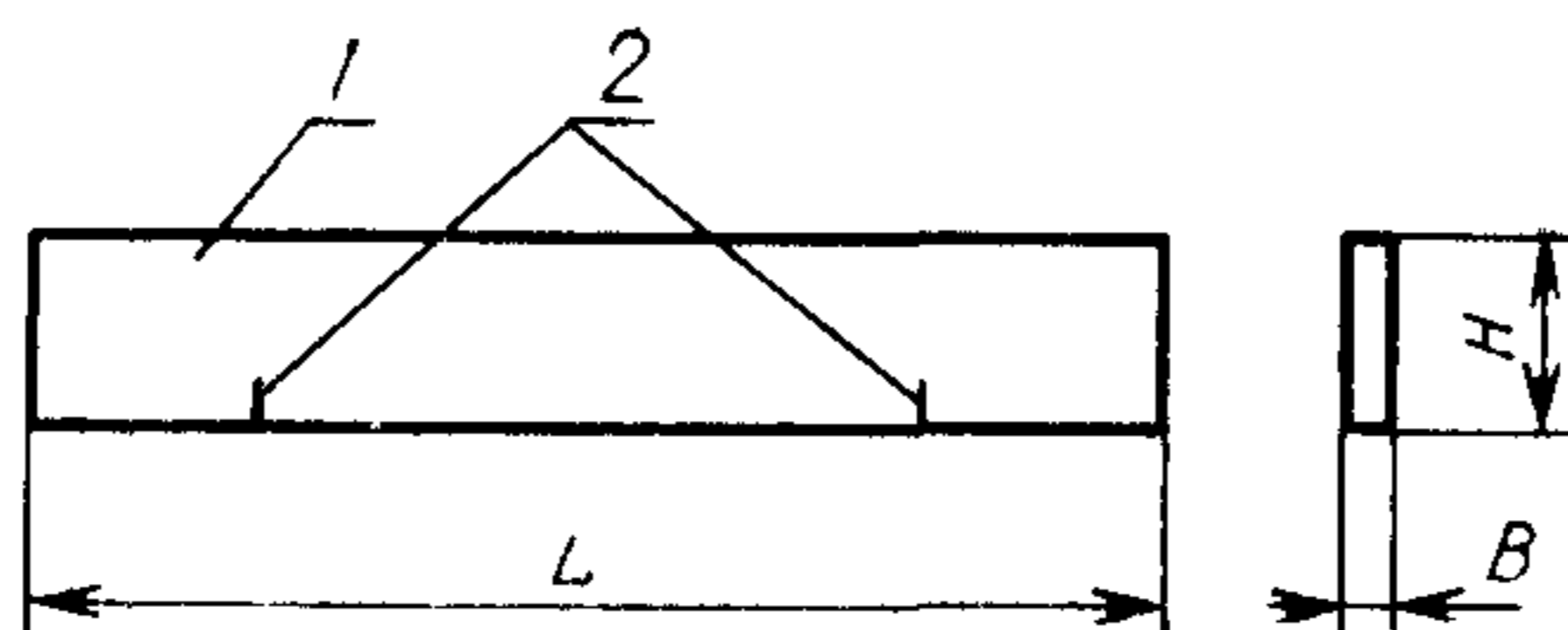
1 рабочая поверхность 2 риски отмечающие точки наименьшего прогиба
