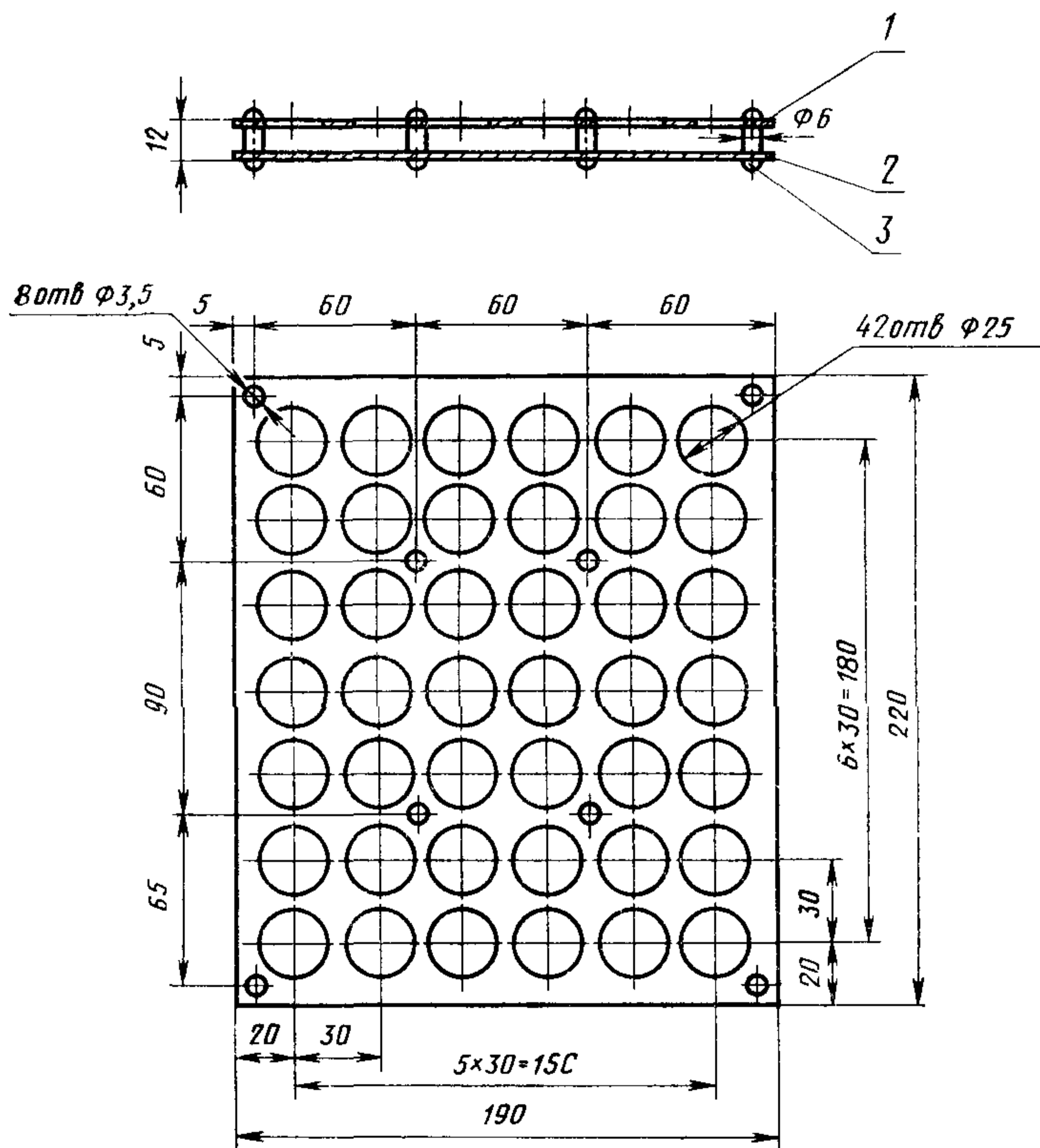
Штатив для тиглей
