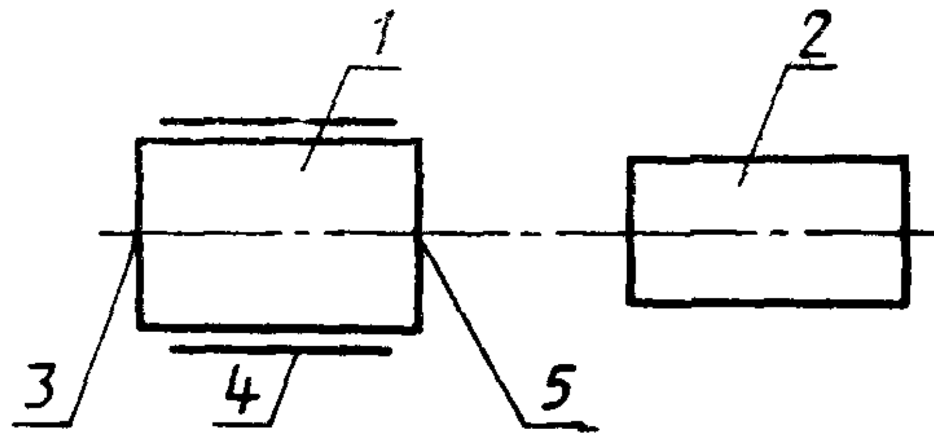
1—ЭОП; 2—яркоммер; 3—фотокатод; 4—держатель; 5—экран
