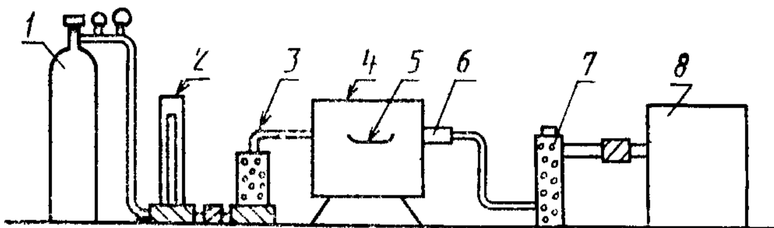
Рисунок 1 — Установка для определения углерода
