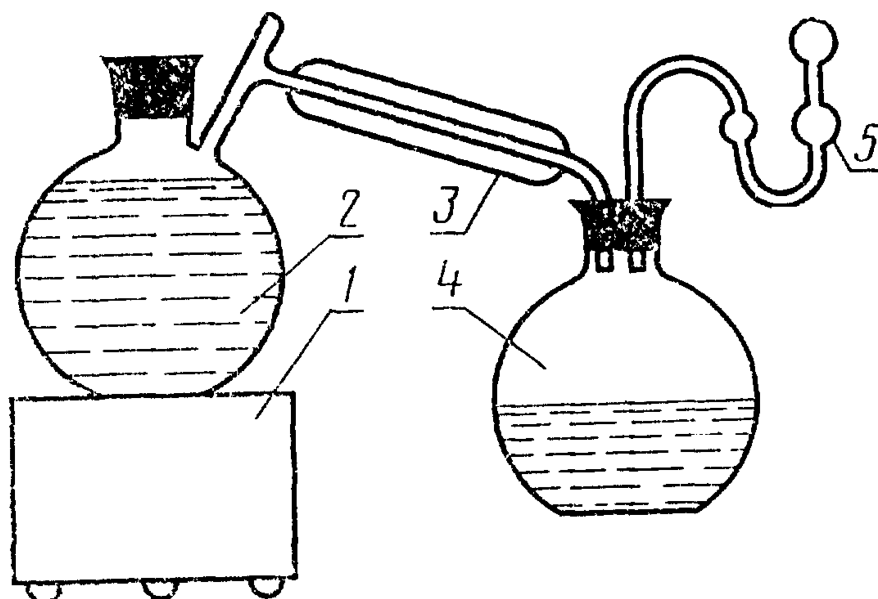
1—электроплитка; 2—дистилляционная колба; 3—холодильник; 4—колба-приемник; 5—предохранительная воронка
