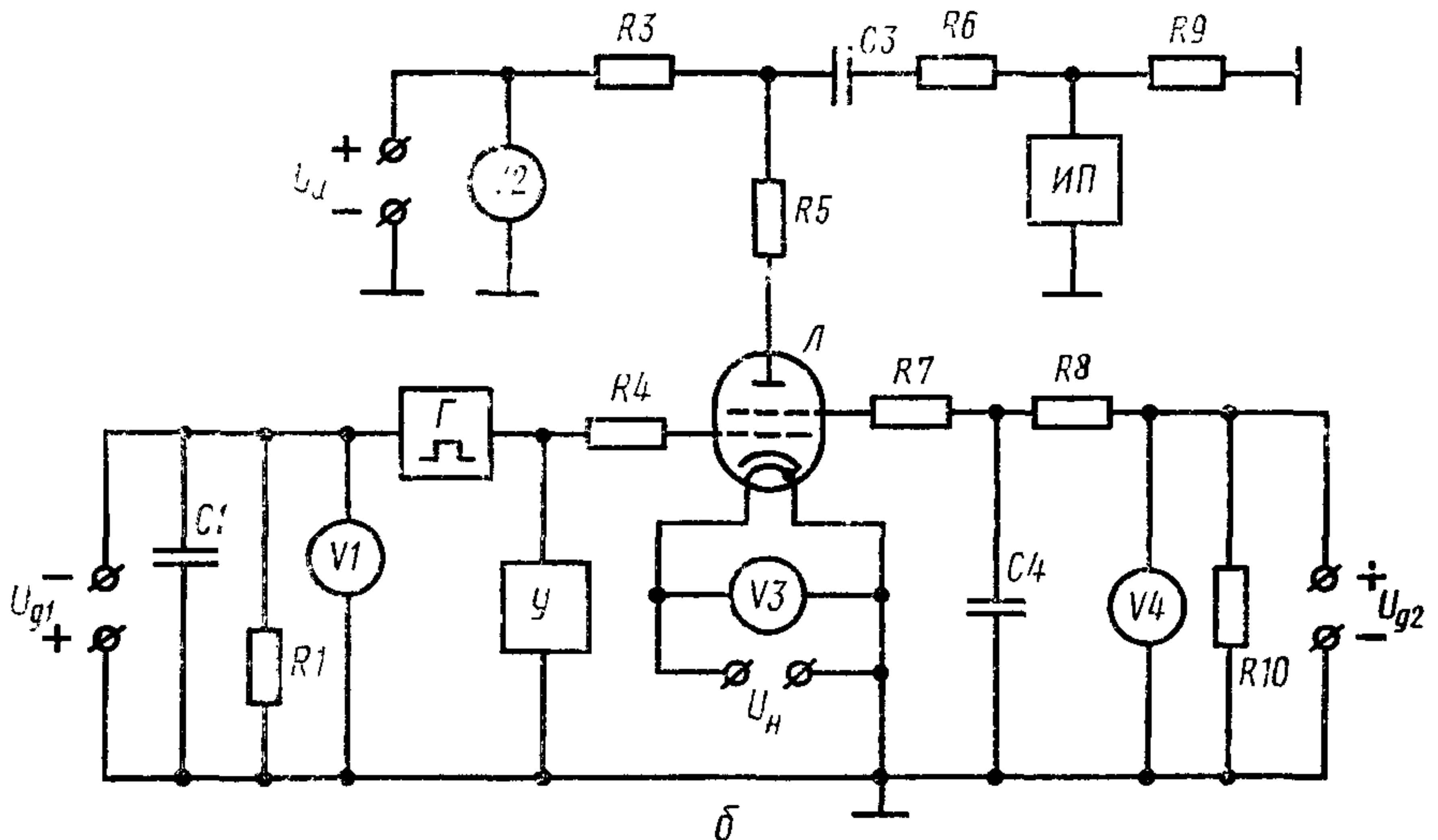
Электрическая схема испытания:
