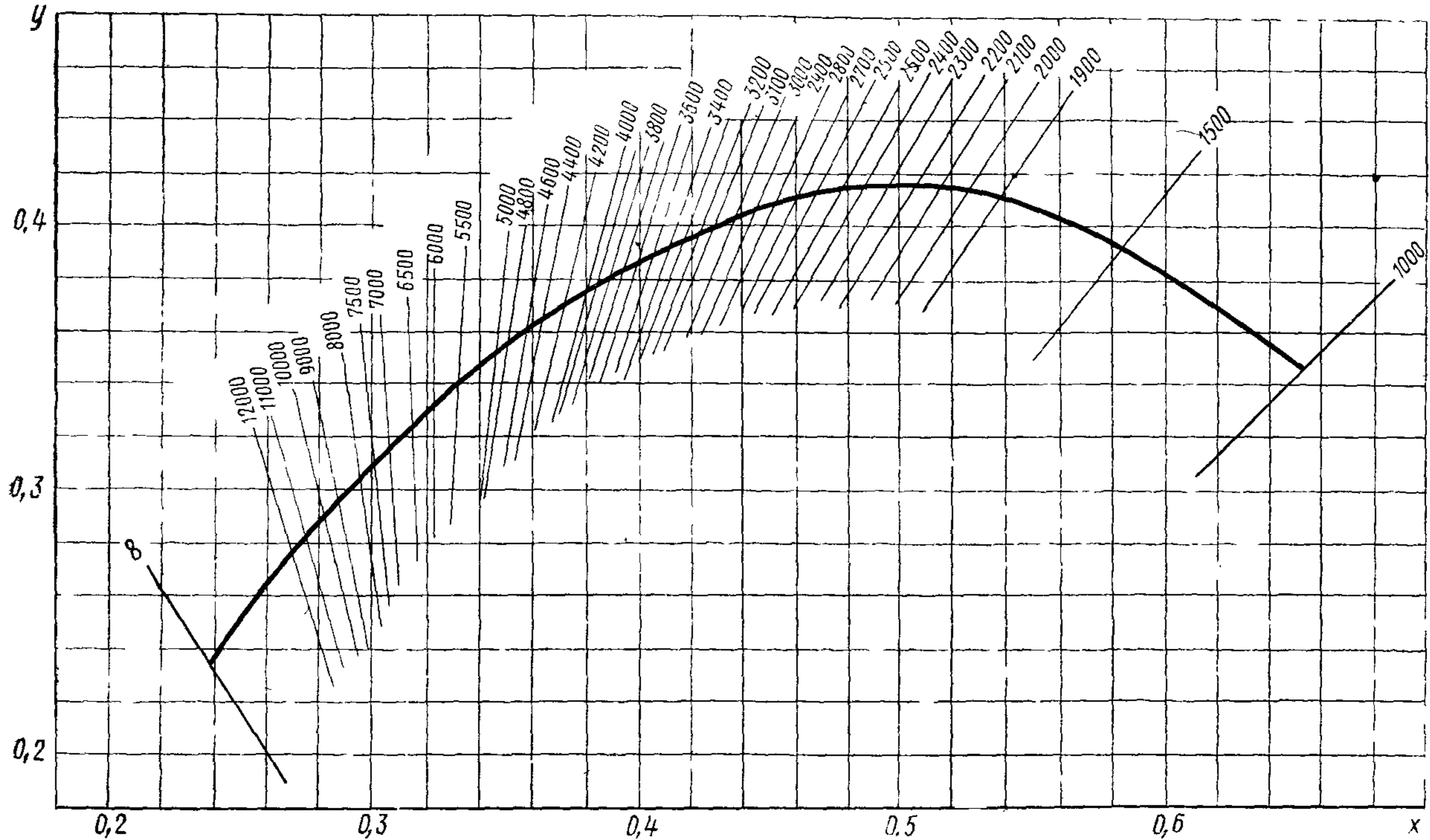
ГРАФИК ДЛЯ ОПРЕДЕЛЕНИЯ ЦВЕТОВОЙ ТЕМПЕРАТУРЫ ЭКРАНОВ КИНЕСКОПОВ ПО КООРДИНАТАМ ЦВЕТНОСТИ ИХ СВЕЧЕНИЯ
