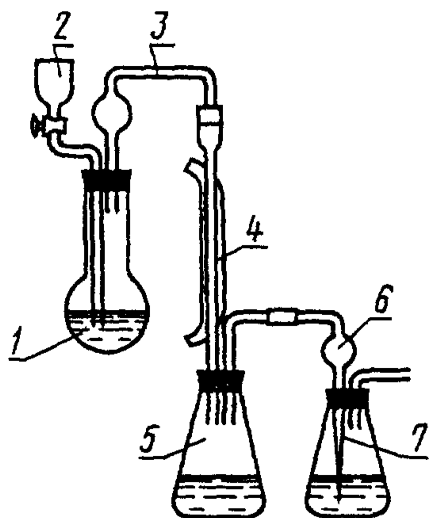
Установка для отгонки мышьяка
