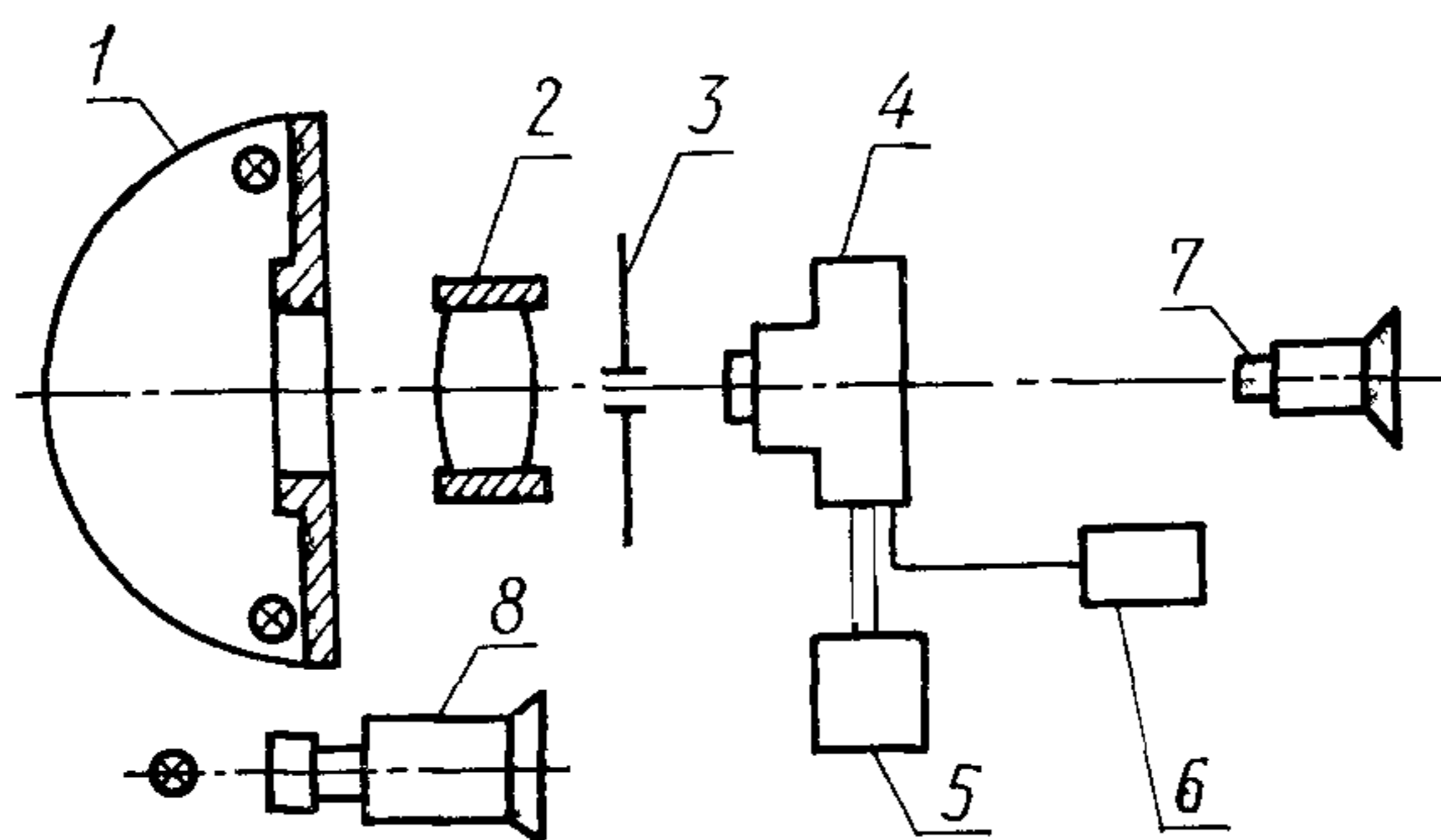
1 — осветитель; 2 — объективодержатель с испытуемым объективом; 3 — измерительная диафрагма, 4 — фотоприемное устройство (ФПУ) 5 — устройство перемещения ФПУ; 6 — регистрирующее устройство; 7 — микроскоп, 8 — коллиматор
