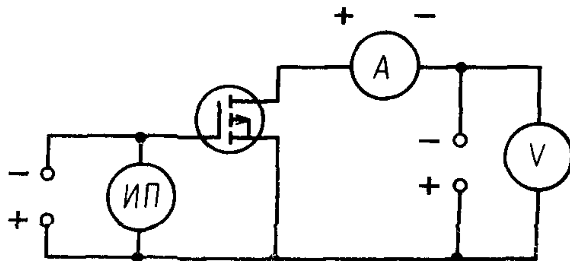
A —измеритель тока; V , ИП —измеритель напряжения.
