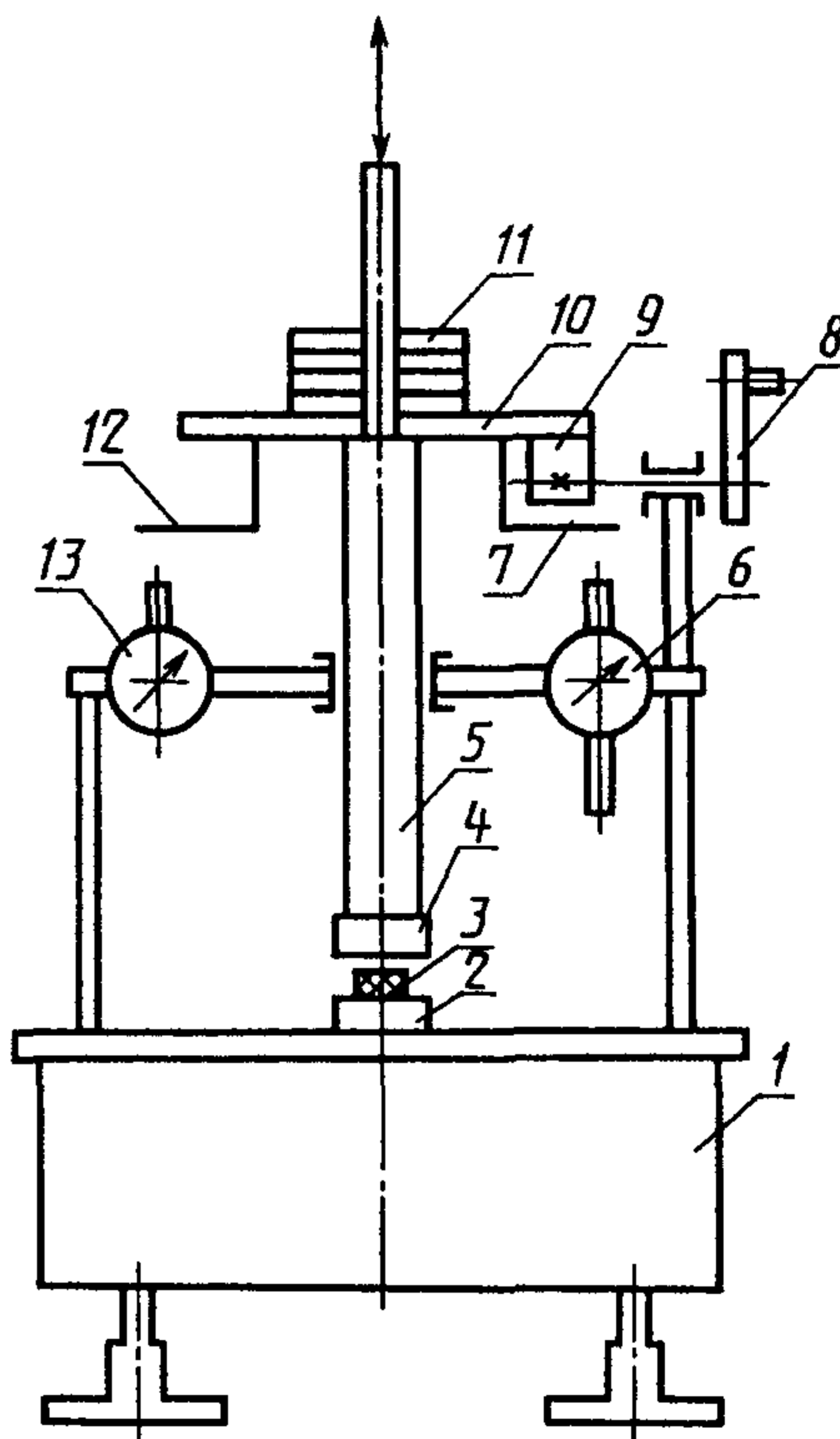
Схема прибора для определения хладотекучести
