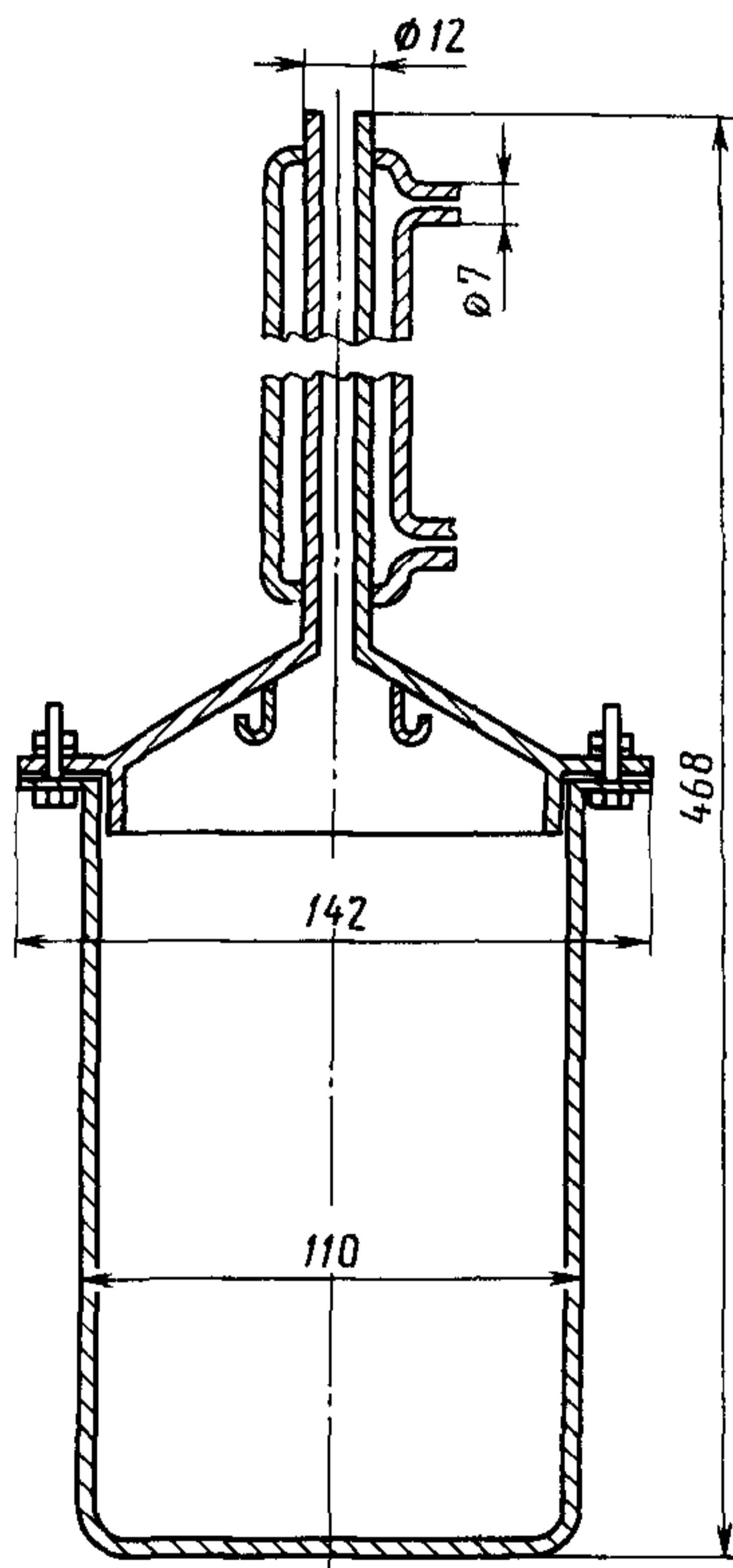
Сосуд с крышкой и холодильником
