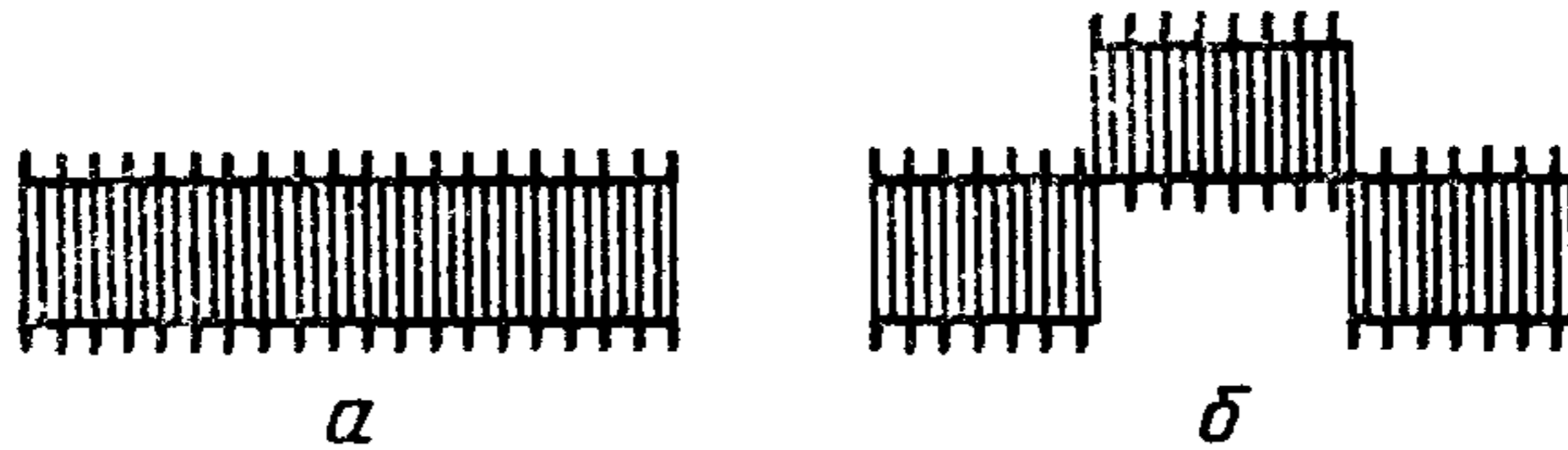
а—шумы в отсутствие сигнала; б—шумы при наличии сигнала в положении, при котором производят отсчет по шкале аттенюатора
