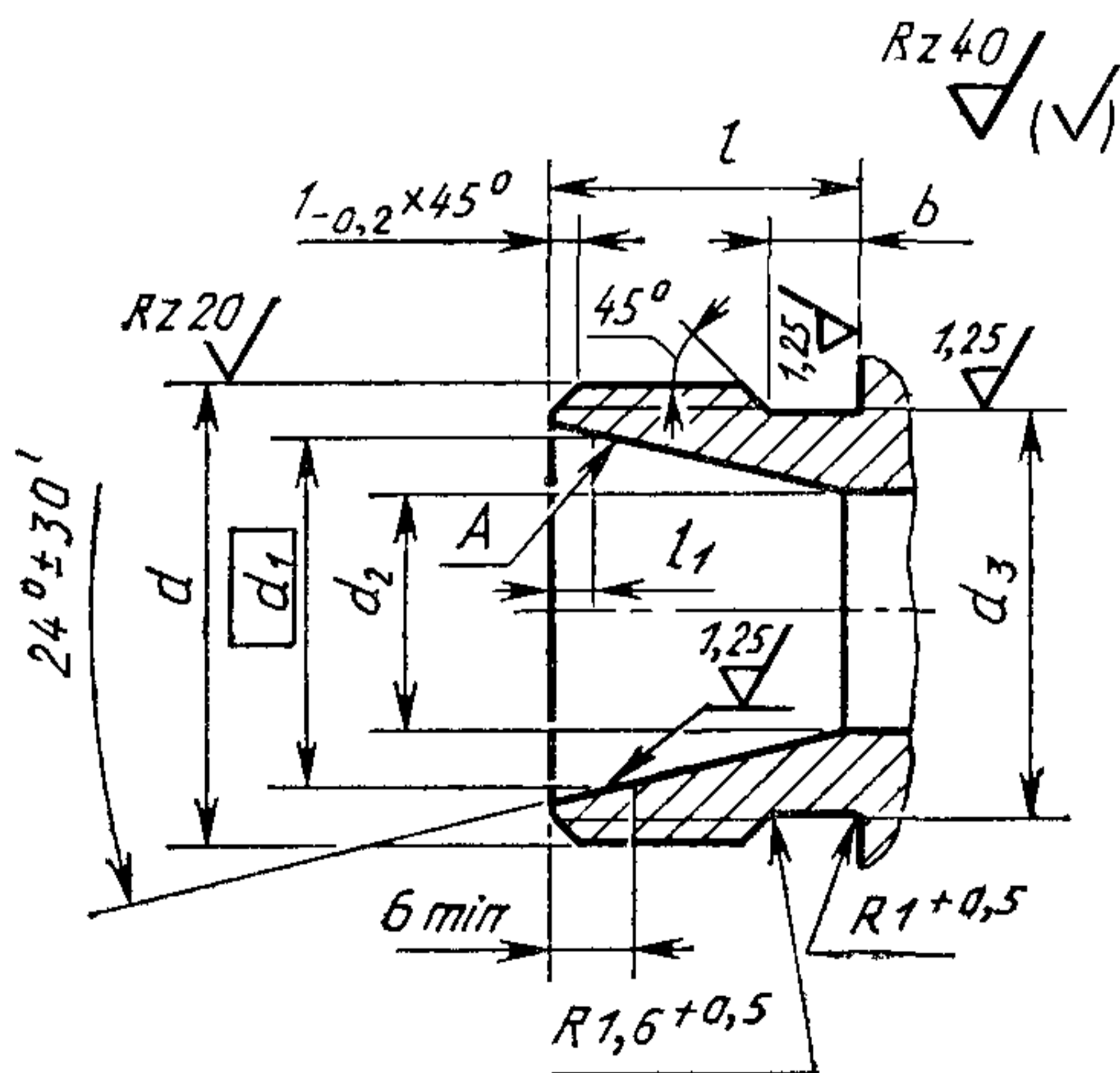
Конструкция и размеры соединительной части штуцеров клапанов типа 7
