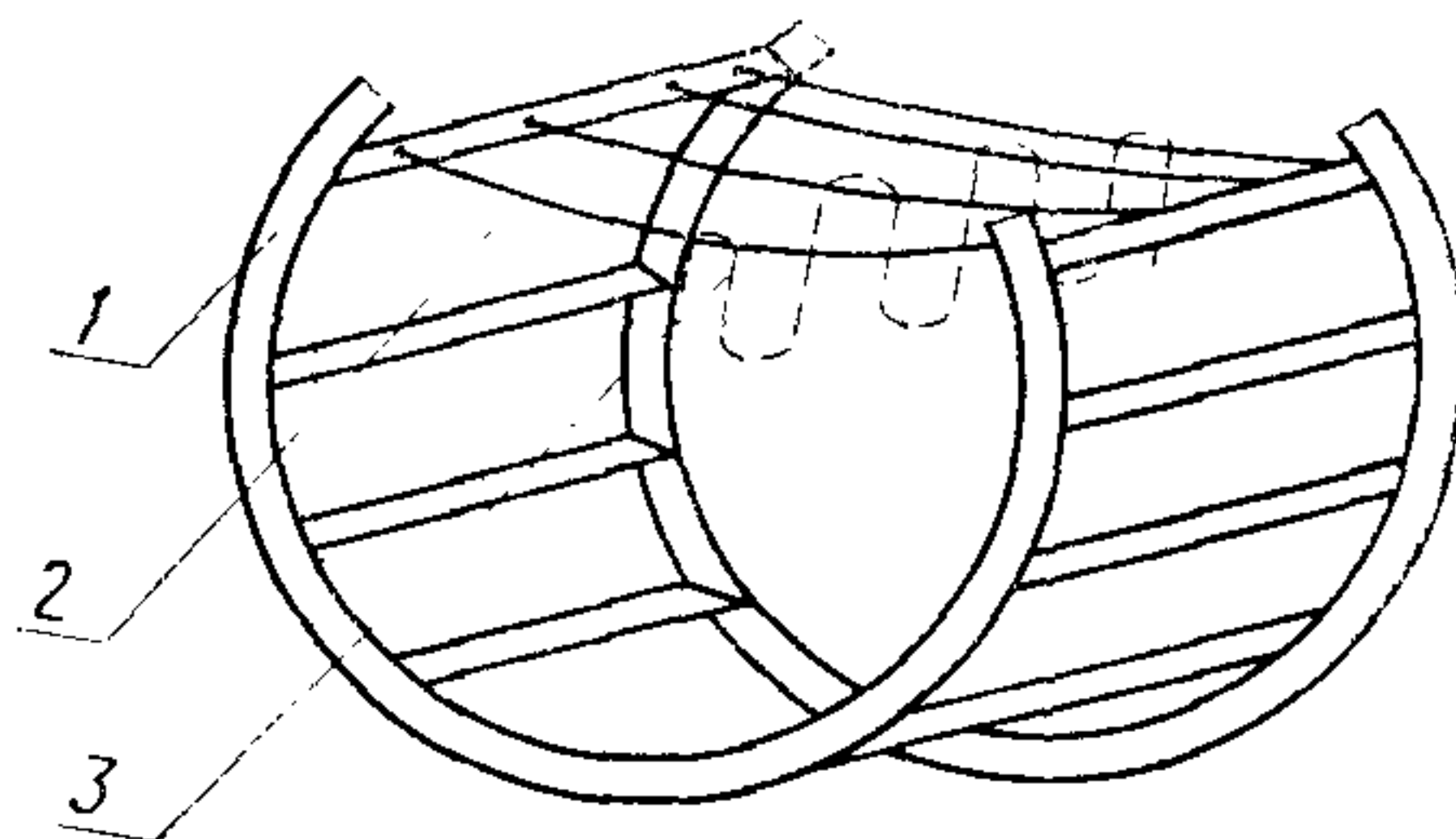
1—металлическая рамка; 2—натянутые термостойкие нити; 3—испытуемая нить в свободном состоянии.
