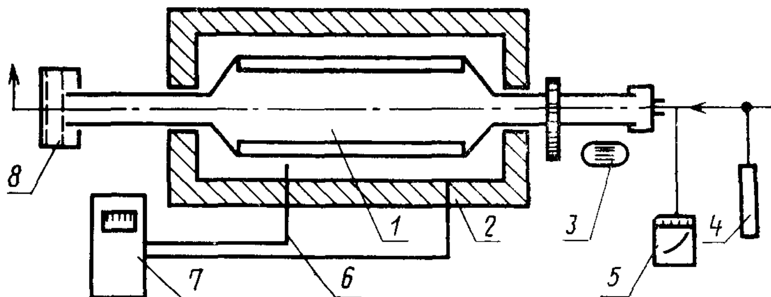
Установка для определения прочности при восстановлении
