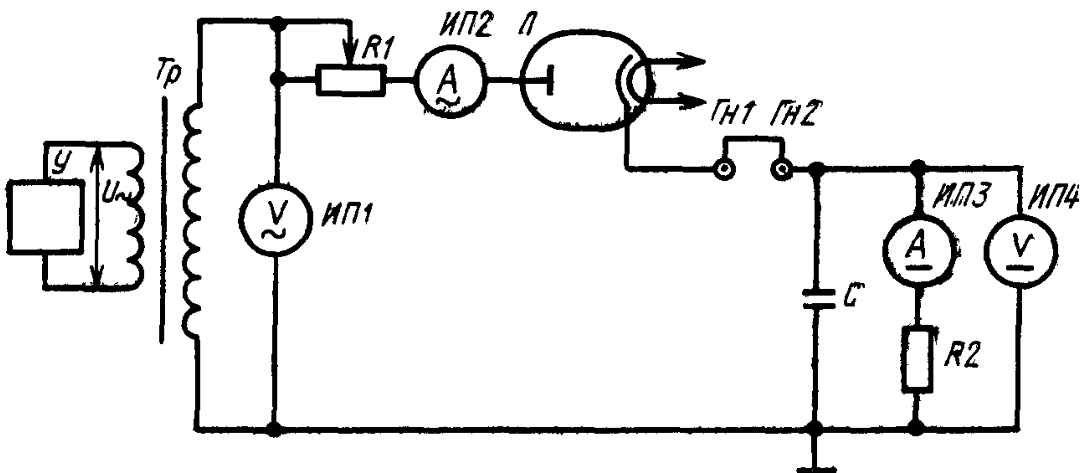
Принципиальная электрическая схема испытания одноанодных выпрямительных ламп на вентиляную прочность
