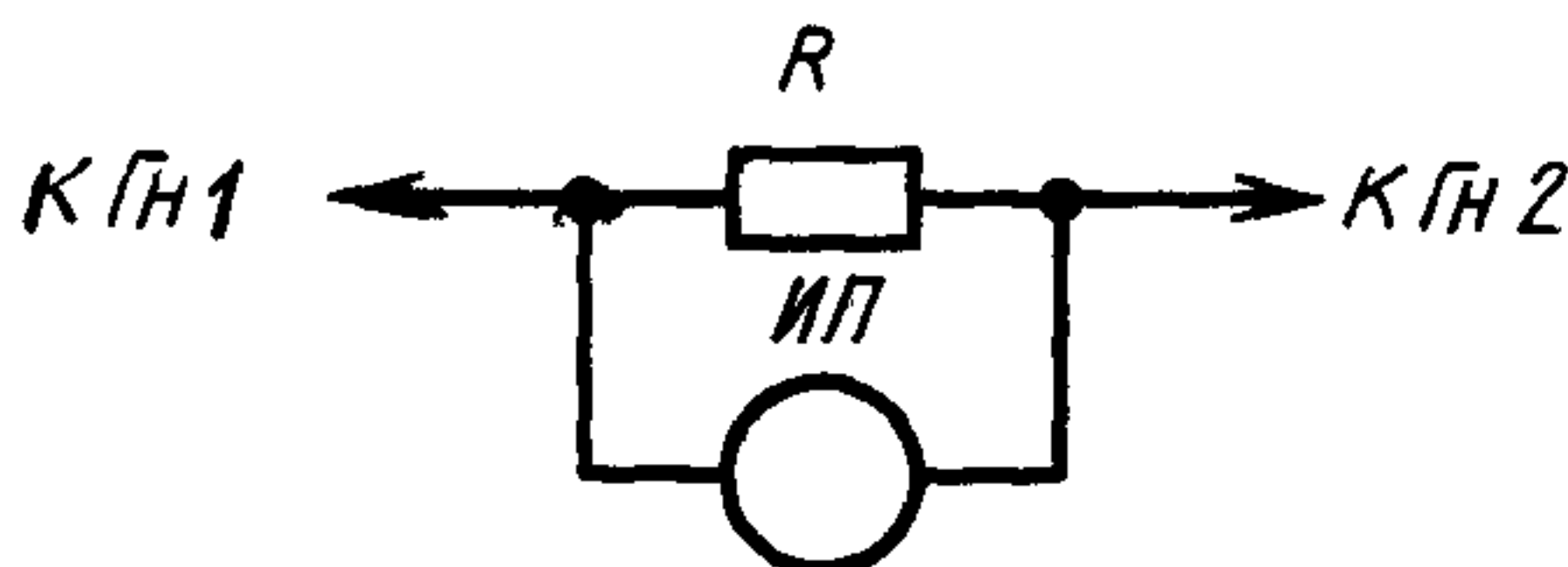
Принципиальная электрическая схема устройства измерения амплитуды импульса
