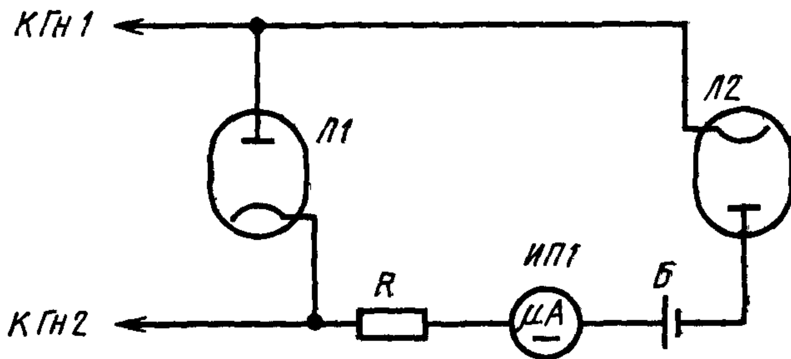
Принципиальная электрическая схема устройства измерения обратного тока
