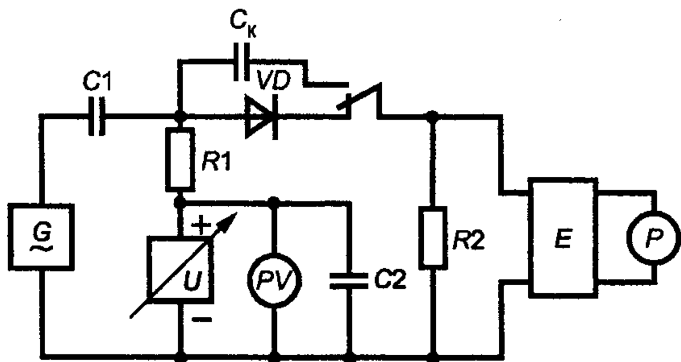
G — генератор переменного напряжения; C_1, C_2 — конденсаторы; C_k — калибровочный конденсатор; VD — проверяемый диод; R_1, R_2 — резисторы; U — регулируемый блок смещения; PV — измеритель напряжения; E — селективный усилитель; P — измерительный прибор
