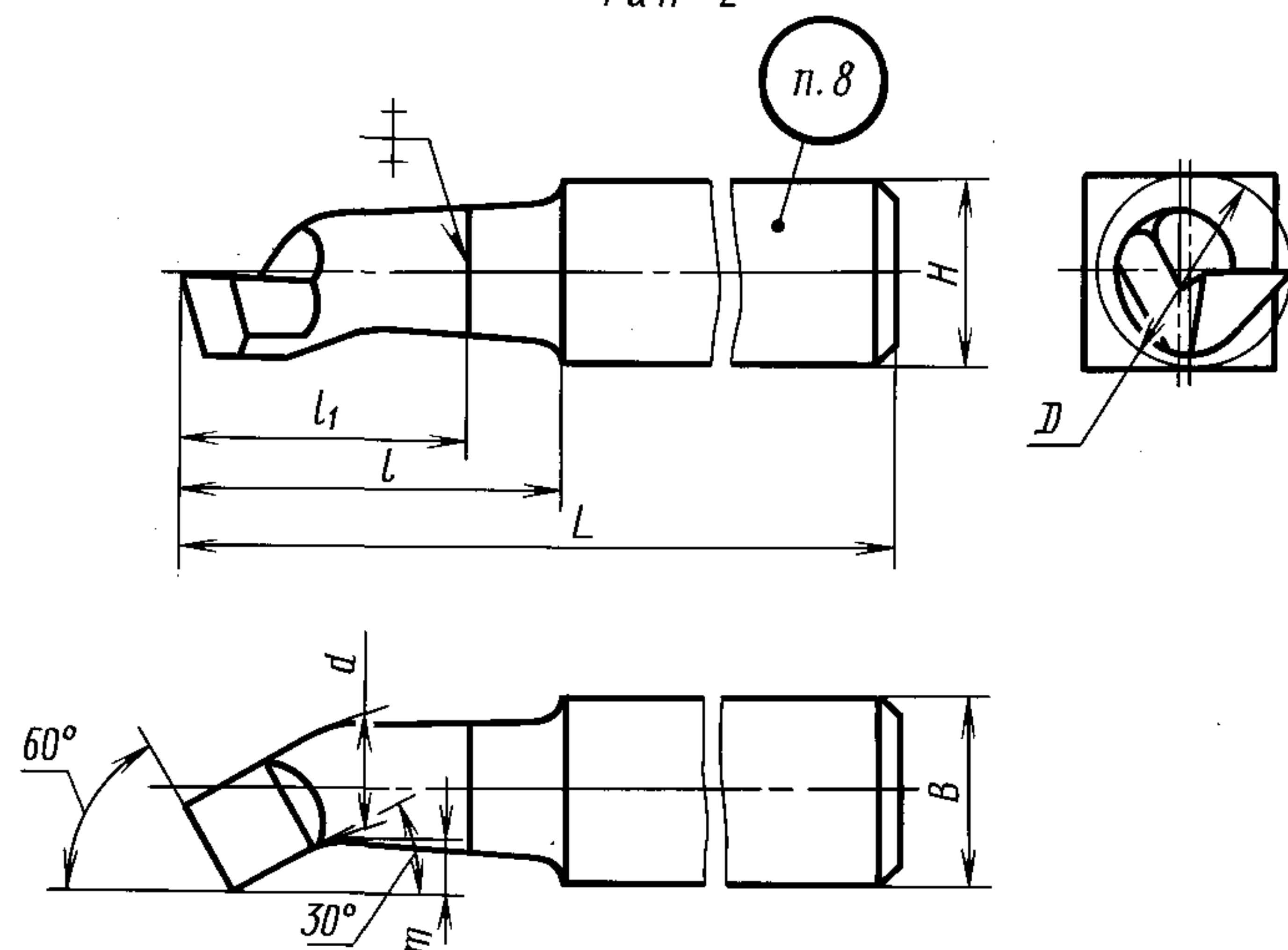
Черт. 2
