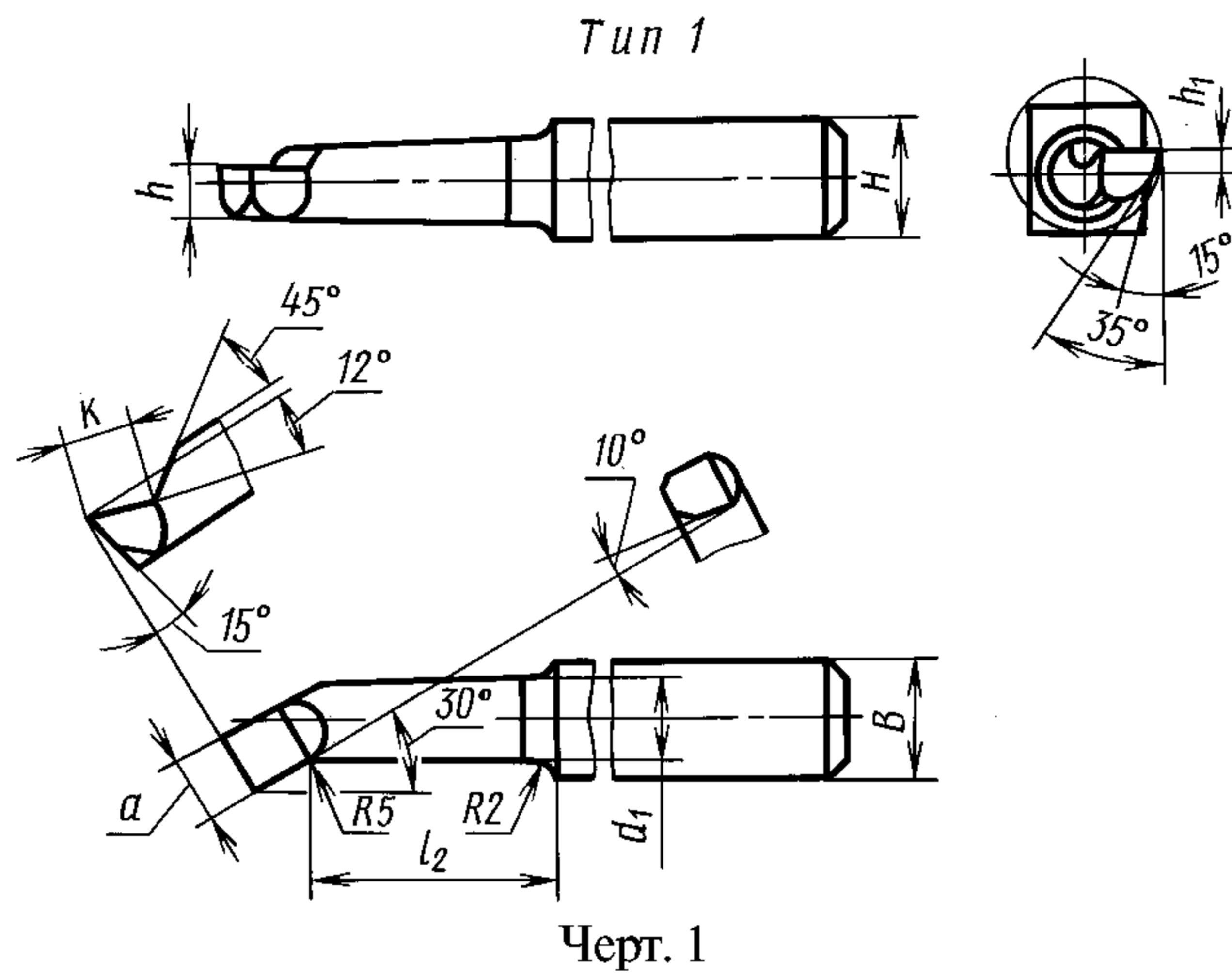
Размеры, мм
