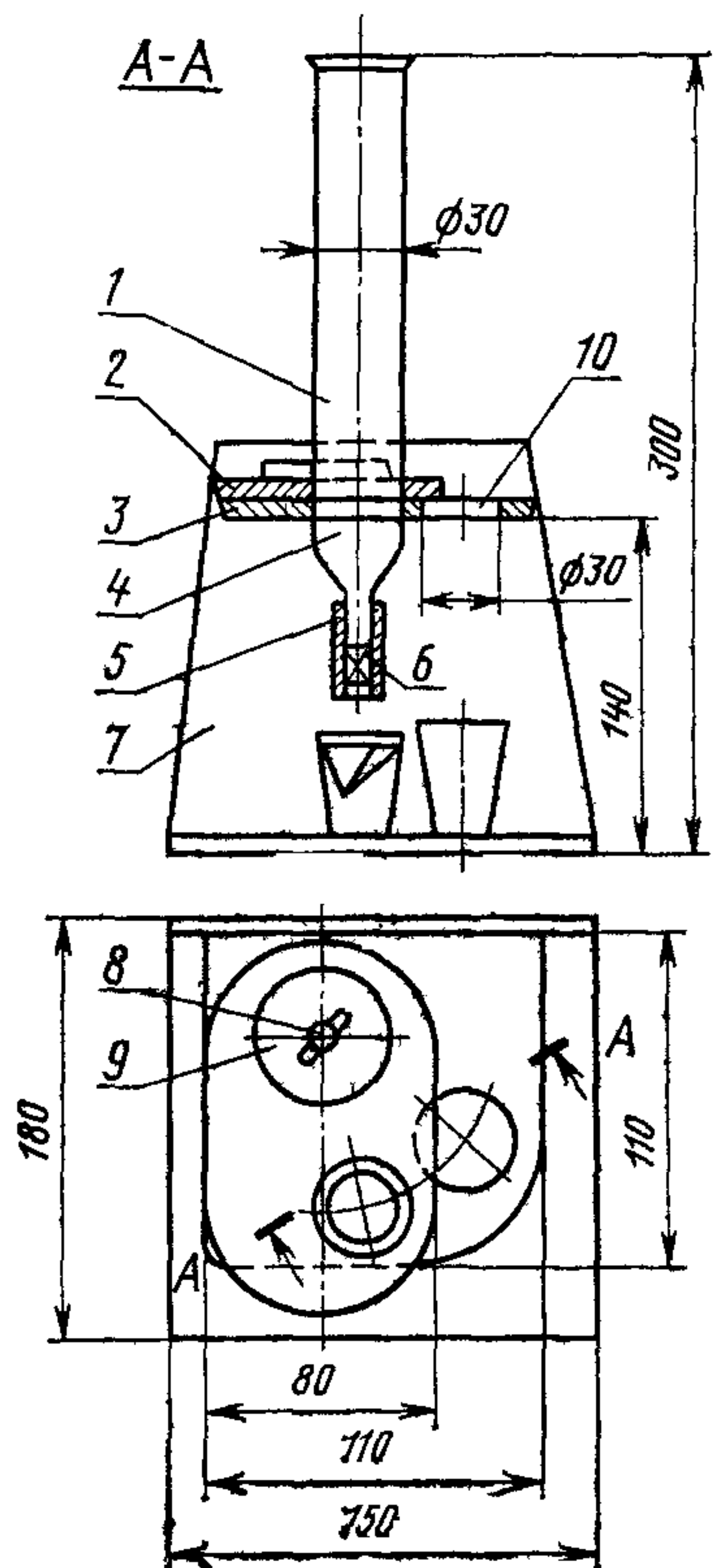
Прибор для определения содержания минеральных примесей
