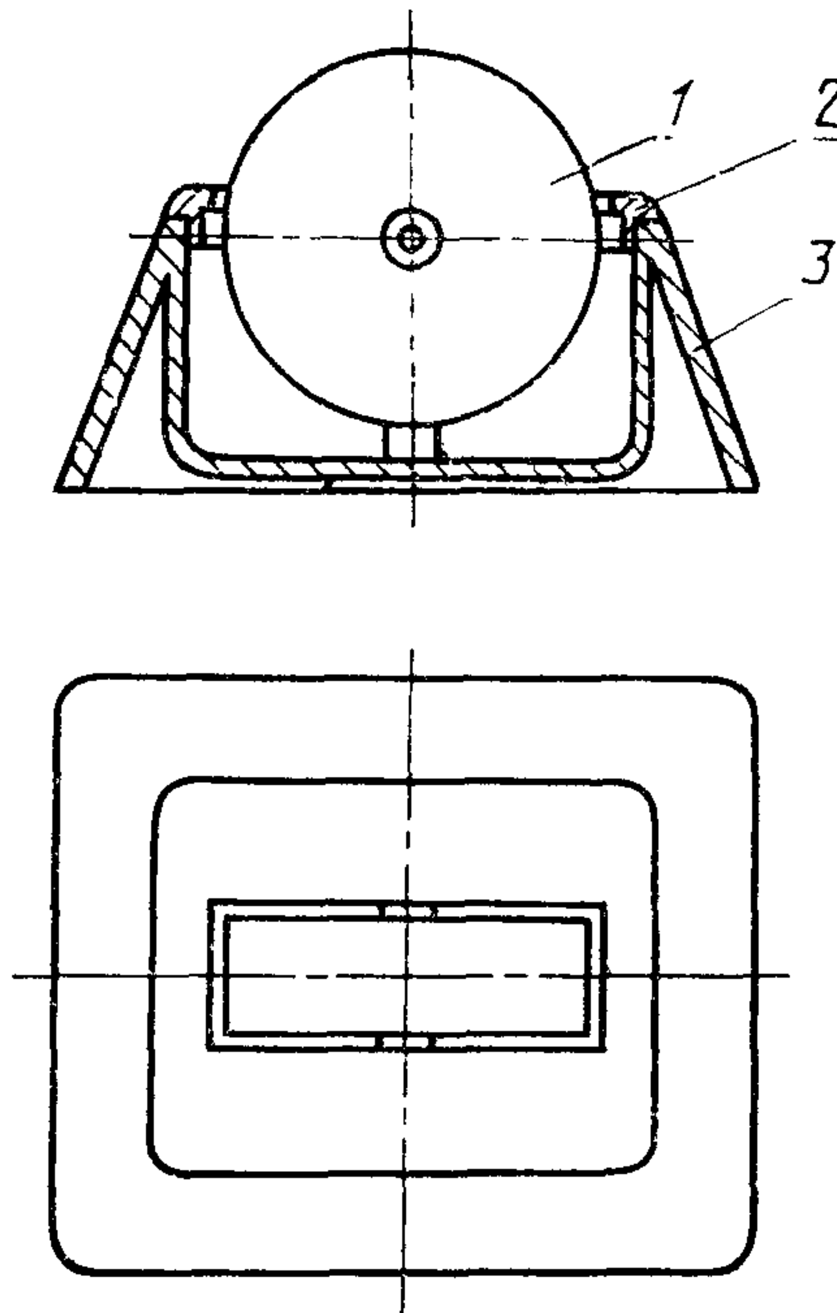
1 — валик; 2 — крышка; 3 — корпус
