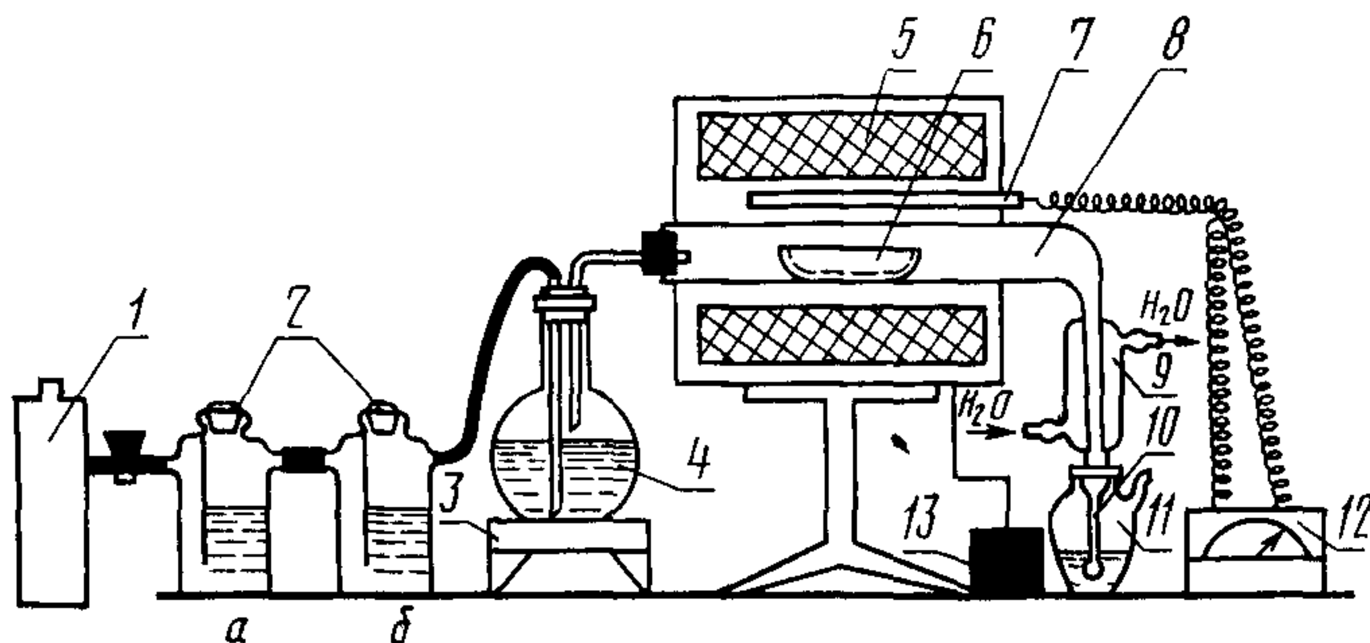
1 — баллон с азотом 2 — промывные склянки 3 — элскгропитка 4 — парообразователь 5 — трубка лодка 6 — кварцевая лодочка 7 — термопара 8 — кварцевая трубка 9 — холодильник 10 — отводная трубка с барботером 11 — колба приемник 12 — микровысмер 13 — автотрансформатор
