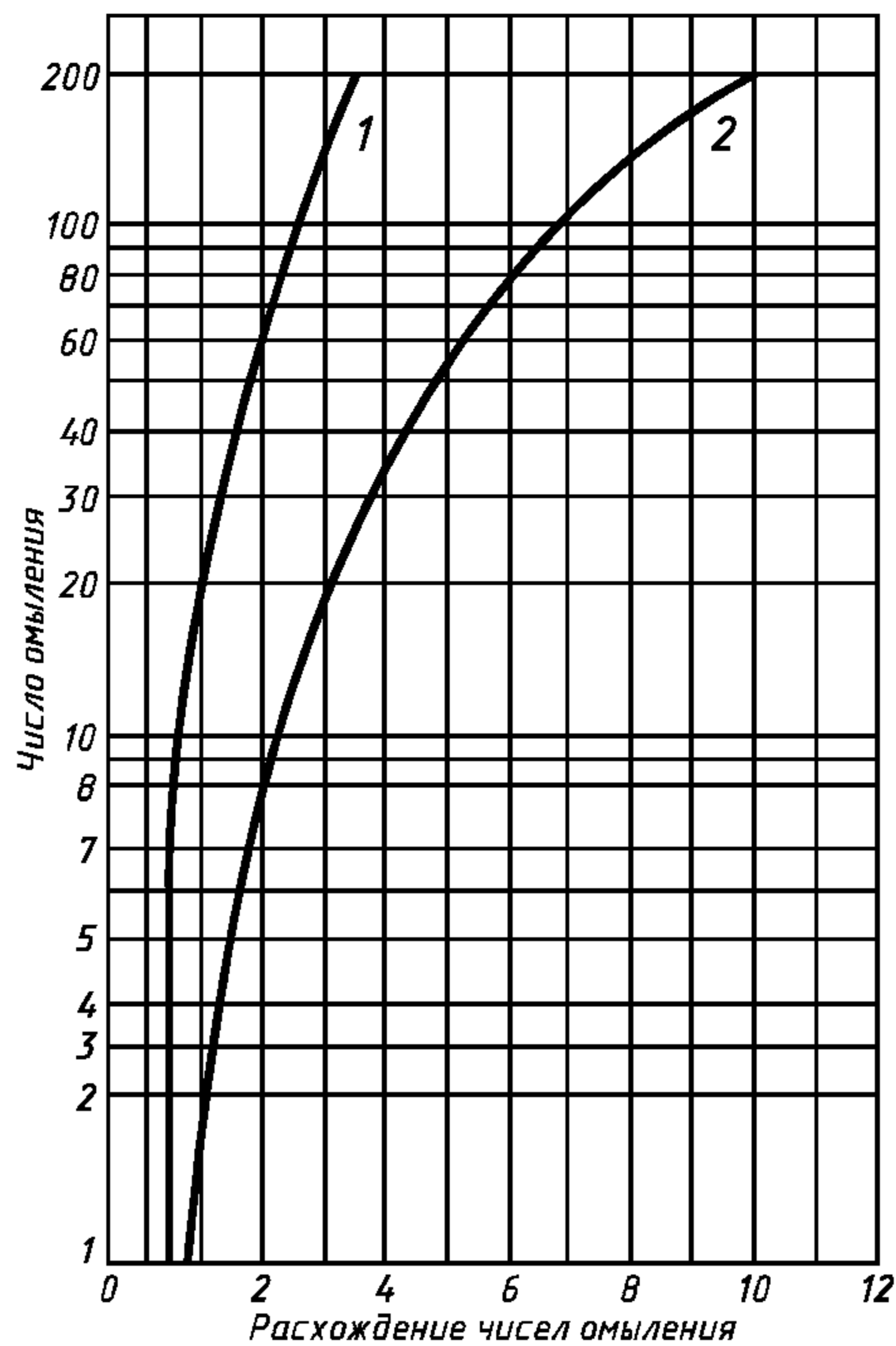
1 — сходимость; 2 — воспроизводимость
