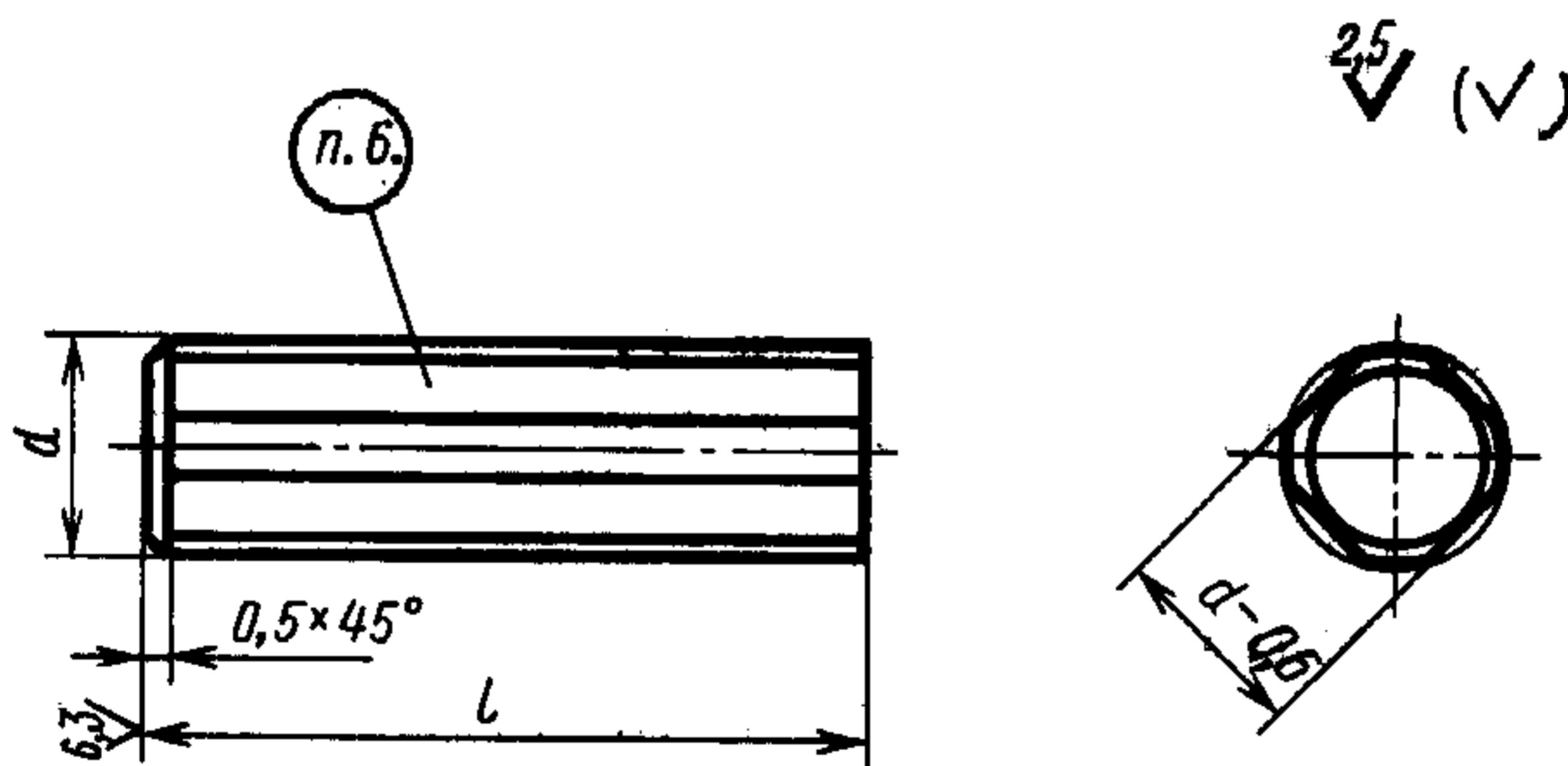
Размеры в мм
