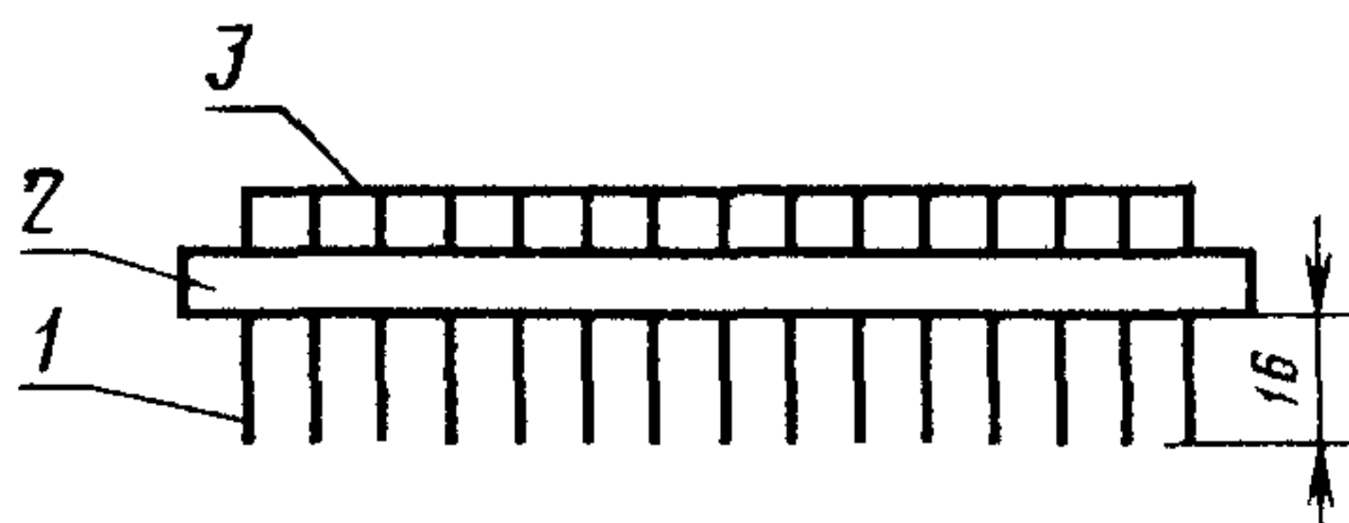
1—игольчатые электроды 2—диск; 3—проводник
