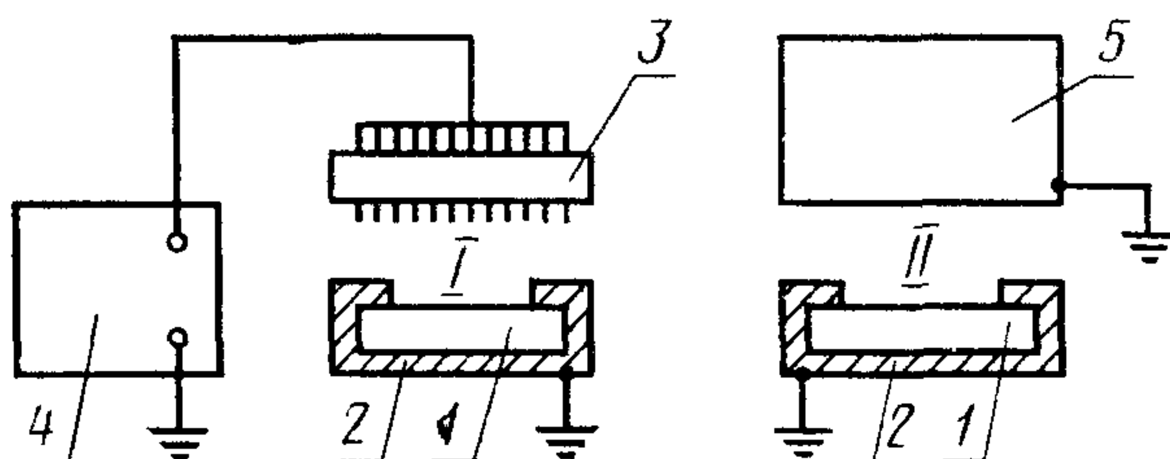
I и II положение образца при электризации и измерении поверхностного заряда соответственно 1—образец; 2—держатель образца, 3—коронирующий электрод, 4—источник высокого напряжения, 5—измеритель электростатического поля
