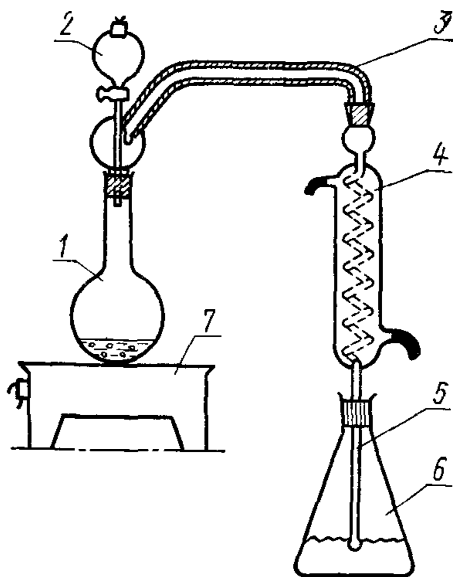
1—дистилляционная колба вместимостью 100 мл, 2—насадка с капельной воронкой, 3—дефлегматор с соединительной трубкой, 4—змеевиковый холодильник, 5—барбатер, 6—пробирка приемник 7—электроплитка
