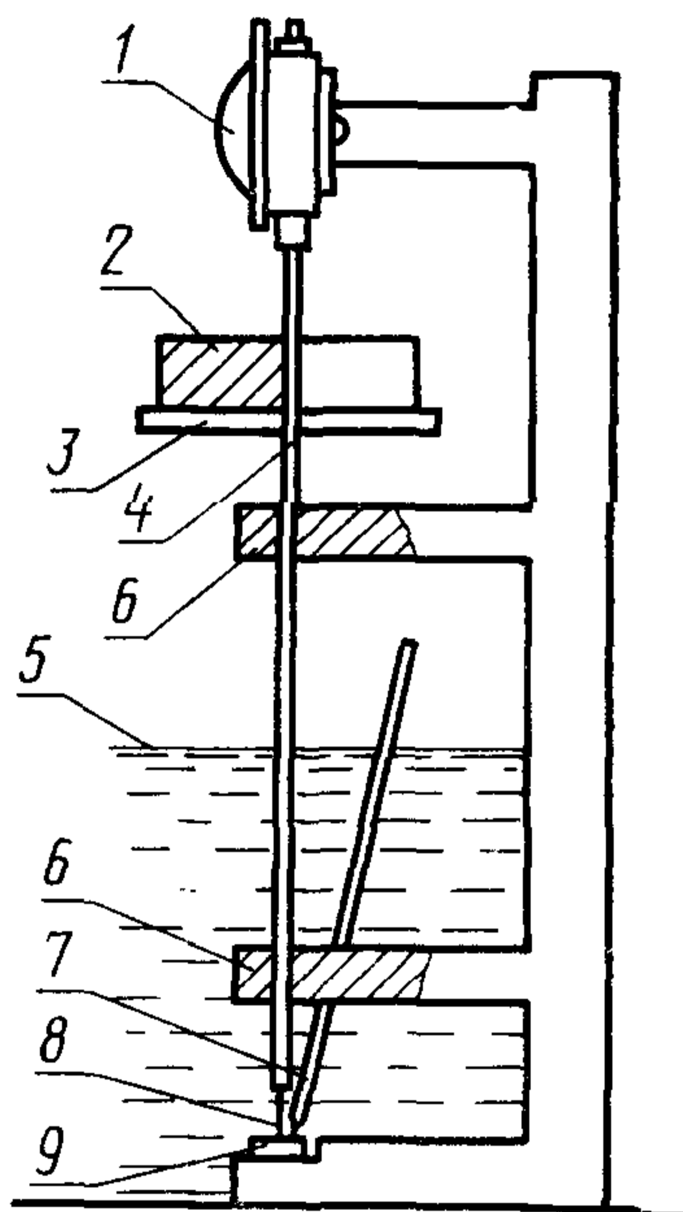
Схема прибора для испытания по Вика
