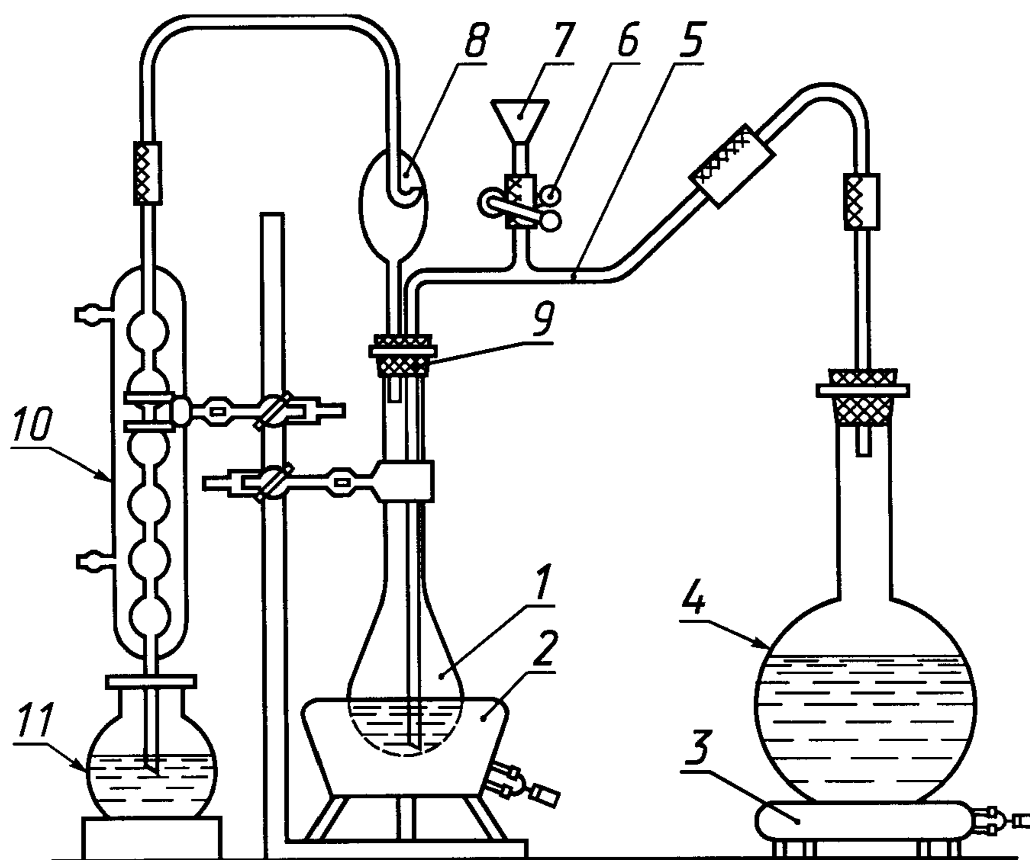
1 — колба Кьельдаля; 2 — колбонагреватель; 3 — электроплитка; 4 — парообразователь; 5 — соединительная трубка; 6 — зажим; 7 — воронка; 8 — каплеуловитель; 9 — пробка; 10 — холодильник; 11 — приемная колба
