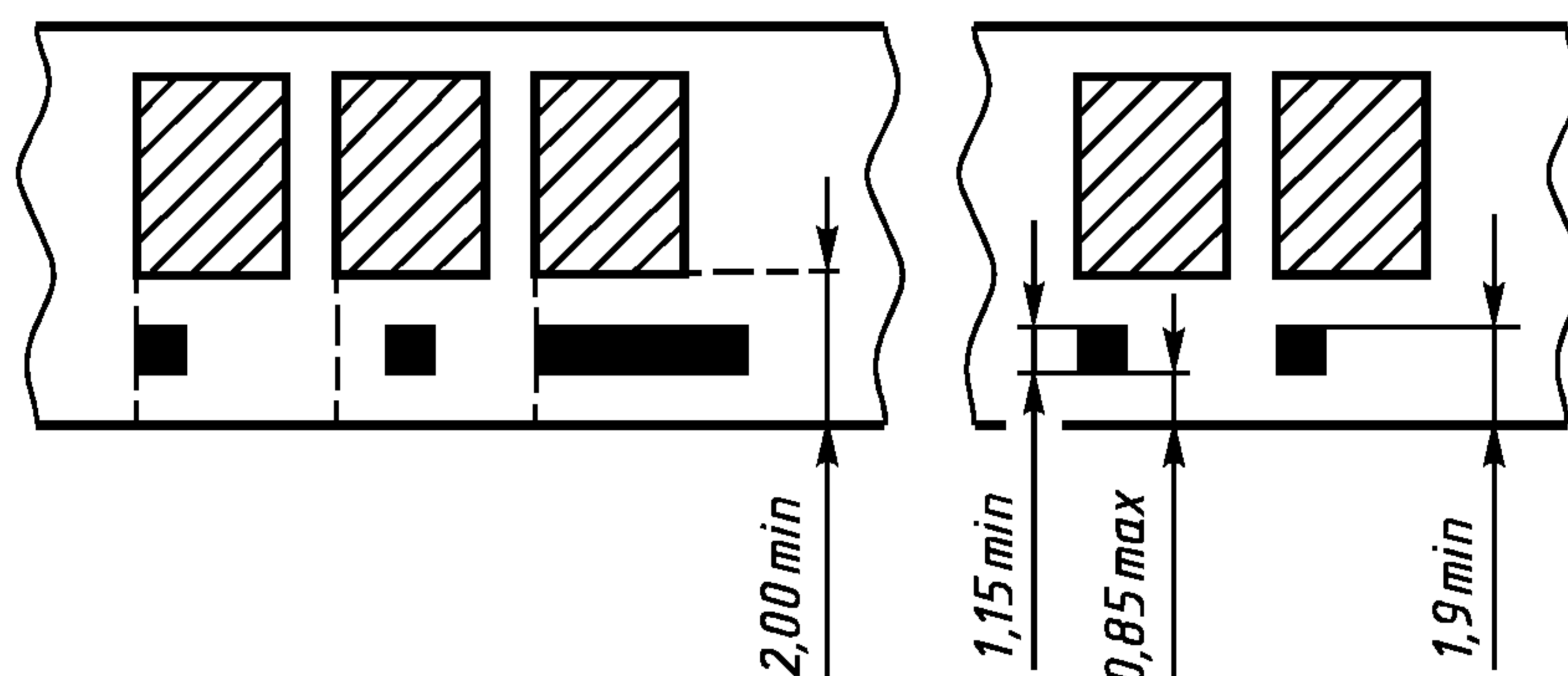
Рисунок 1 — Размещение счетной метки в зоне кодирования
