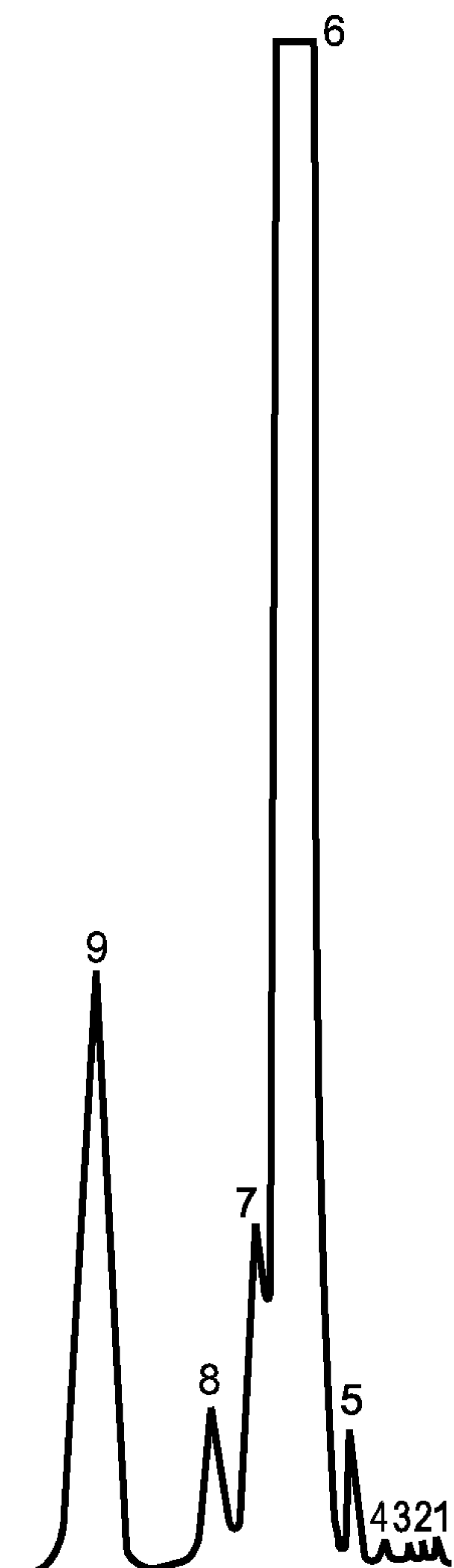
1, 2, 3, 4, 7 — неидентифицированные компоненты; 5 — пентадекан; 6 — гексадекан; 8 — гептадекан; 9 — октадекан (внутренний эталон)
