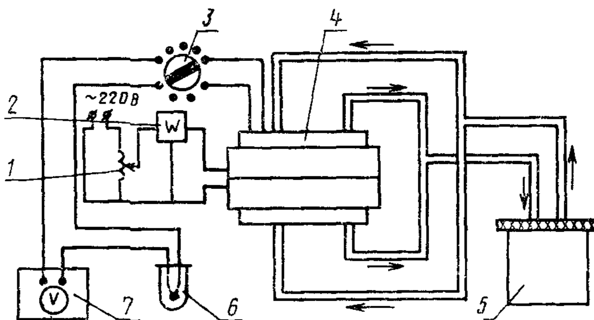
1—автотрансформатор, 2—ваттметр, 3—переключатель тер- мопар 4—рабочая часть 5—термостат 6—холодный тер- мопар 7—электронно цифровой вольтметр
