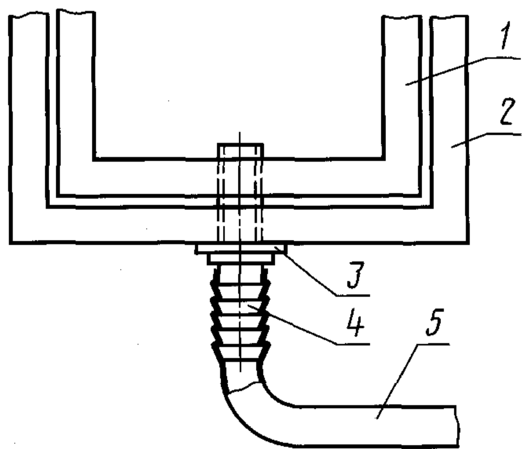
Схема крепления штуцера к рамке
