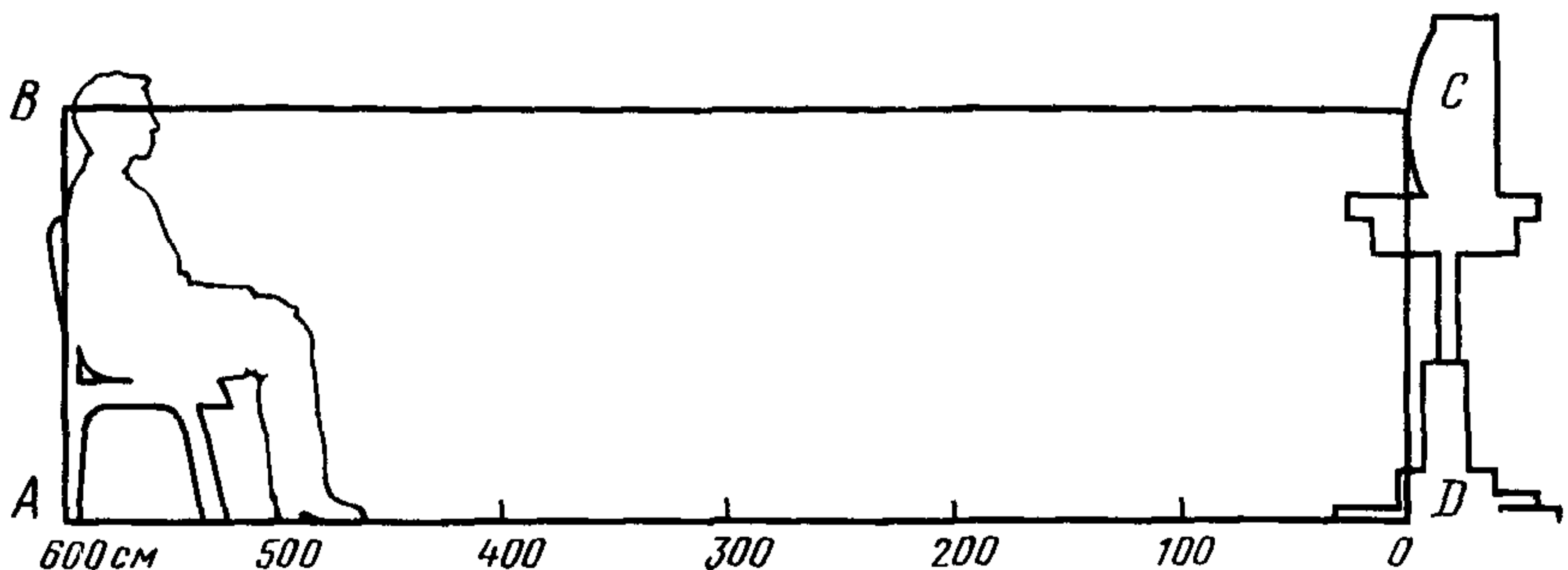
Схема расположения испытателя и прибора типа ПОЗД-2
