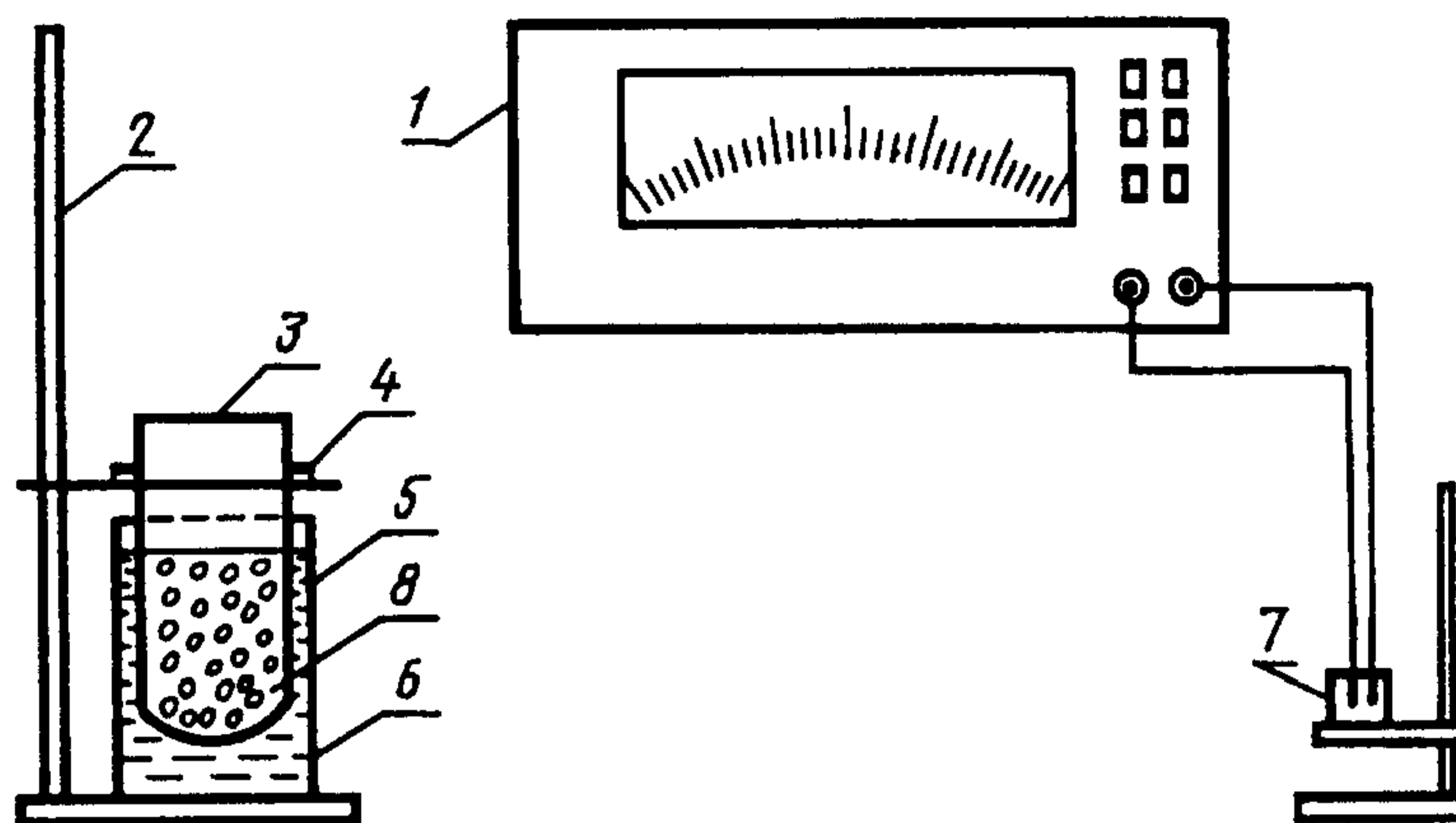
1 — рН-метр-милливольтметр; 2 — штатив с кольцом; 3 — изделие; 4 — стержень; 5 — емкость вместимостью 3 л; 6 — агрессивная жидкость; 7 — стакан для отбора проб; 8 — жидкость в изделии
