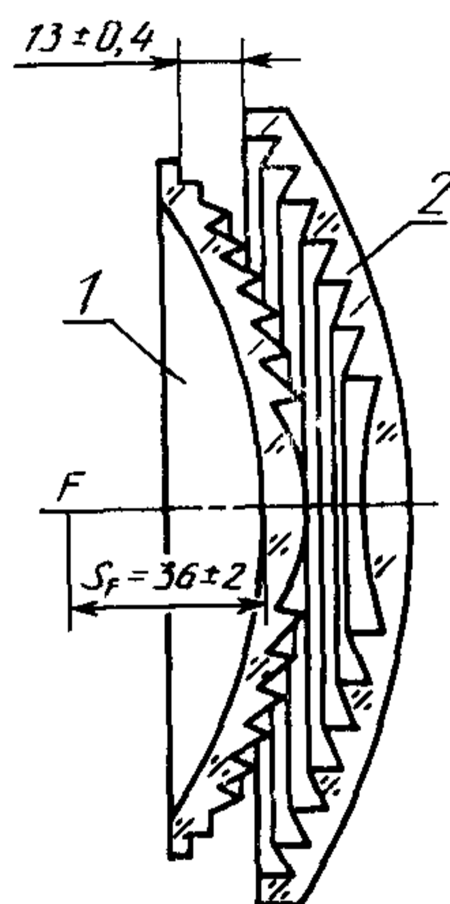
1 — светофильтр-линза СЛ 139 М, 2 — линза ступенчатая ЛС 160
