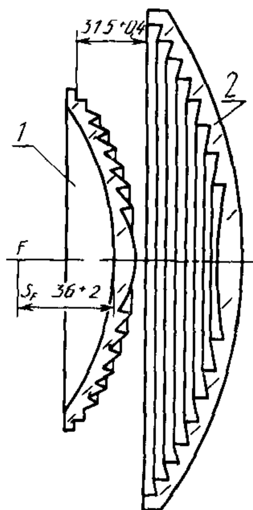
1 — светофильтр-линза СЛ-139 М; 2 — линза ступенчатая ЛС 212
