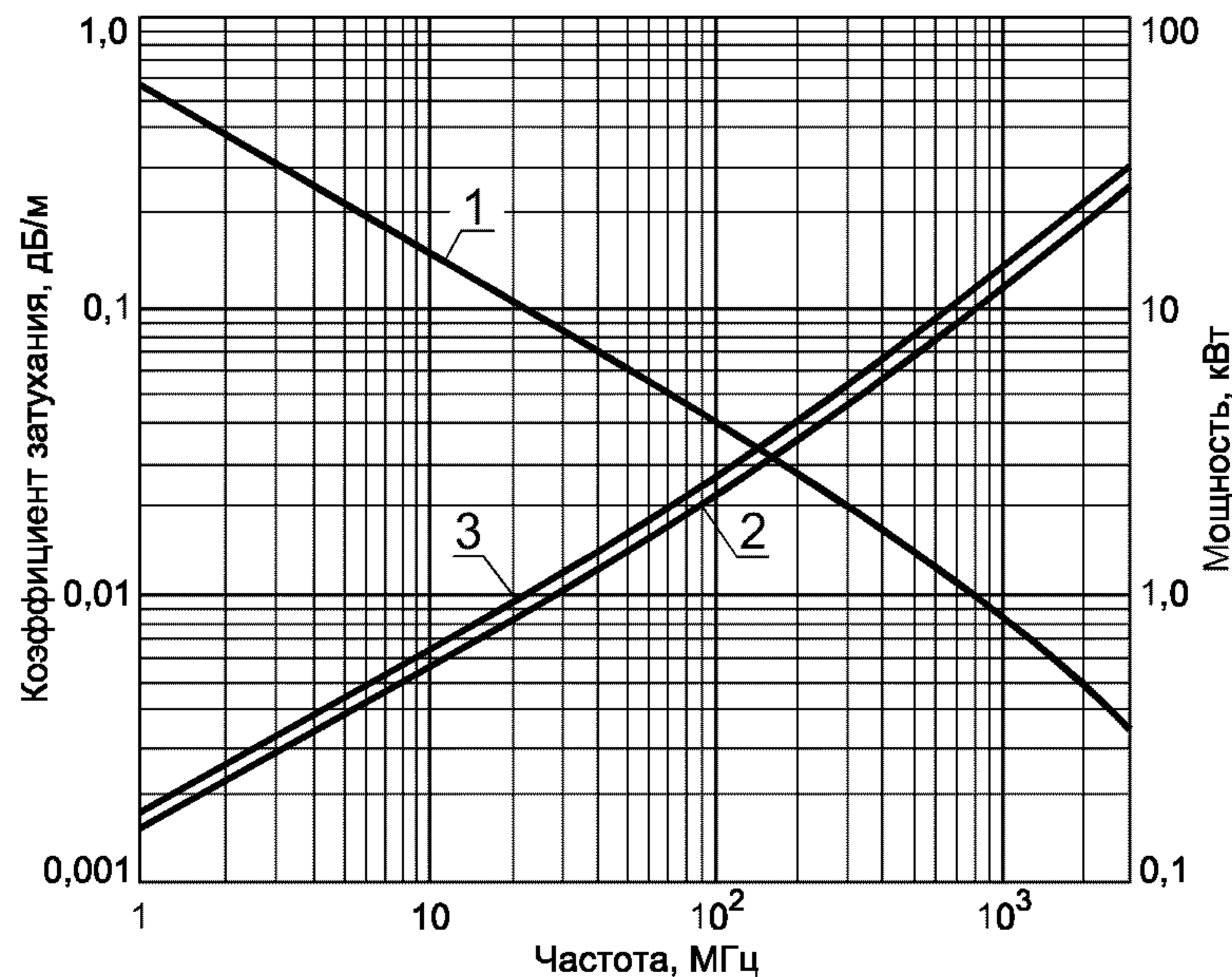
Частотные зависимости
