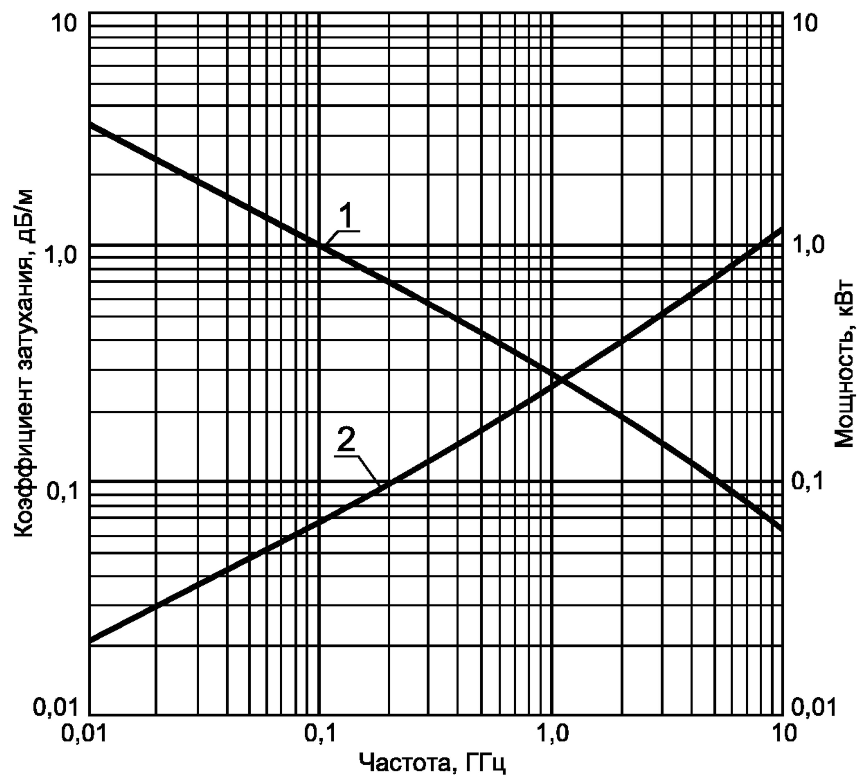
Частотные зависимости
