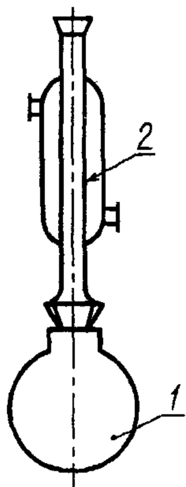
1 — круглодонная колба; 2 — холодильник
