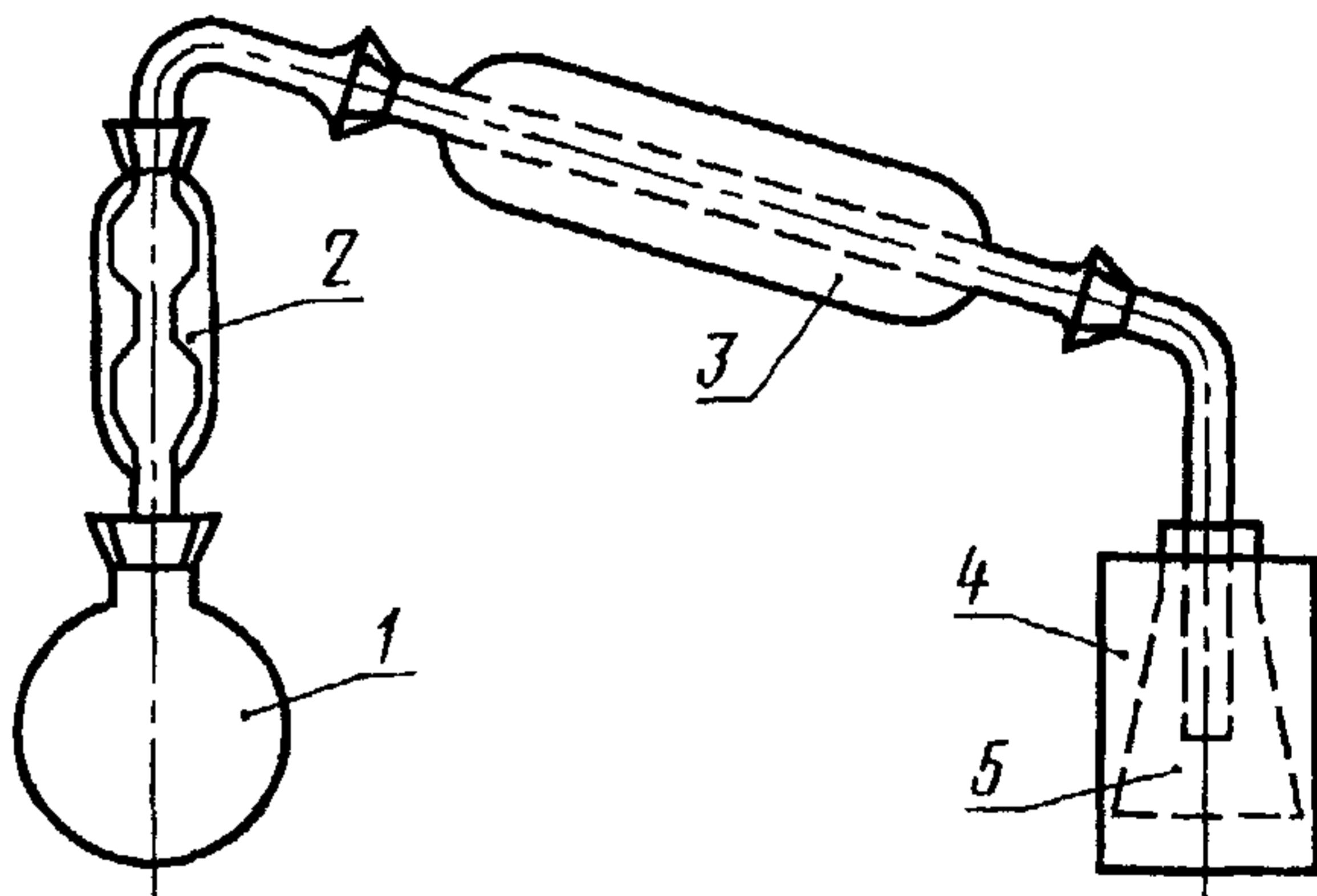
1 — круглодонная колба; 2 — изгиб; 3 — холодильник; 4 — аллонж; 5 — цилиндр
