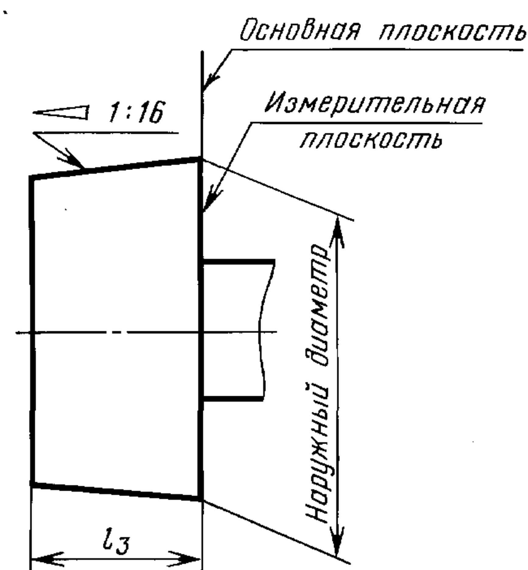
Калибр-пробка К-Г
