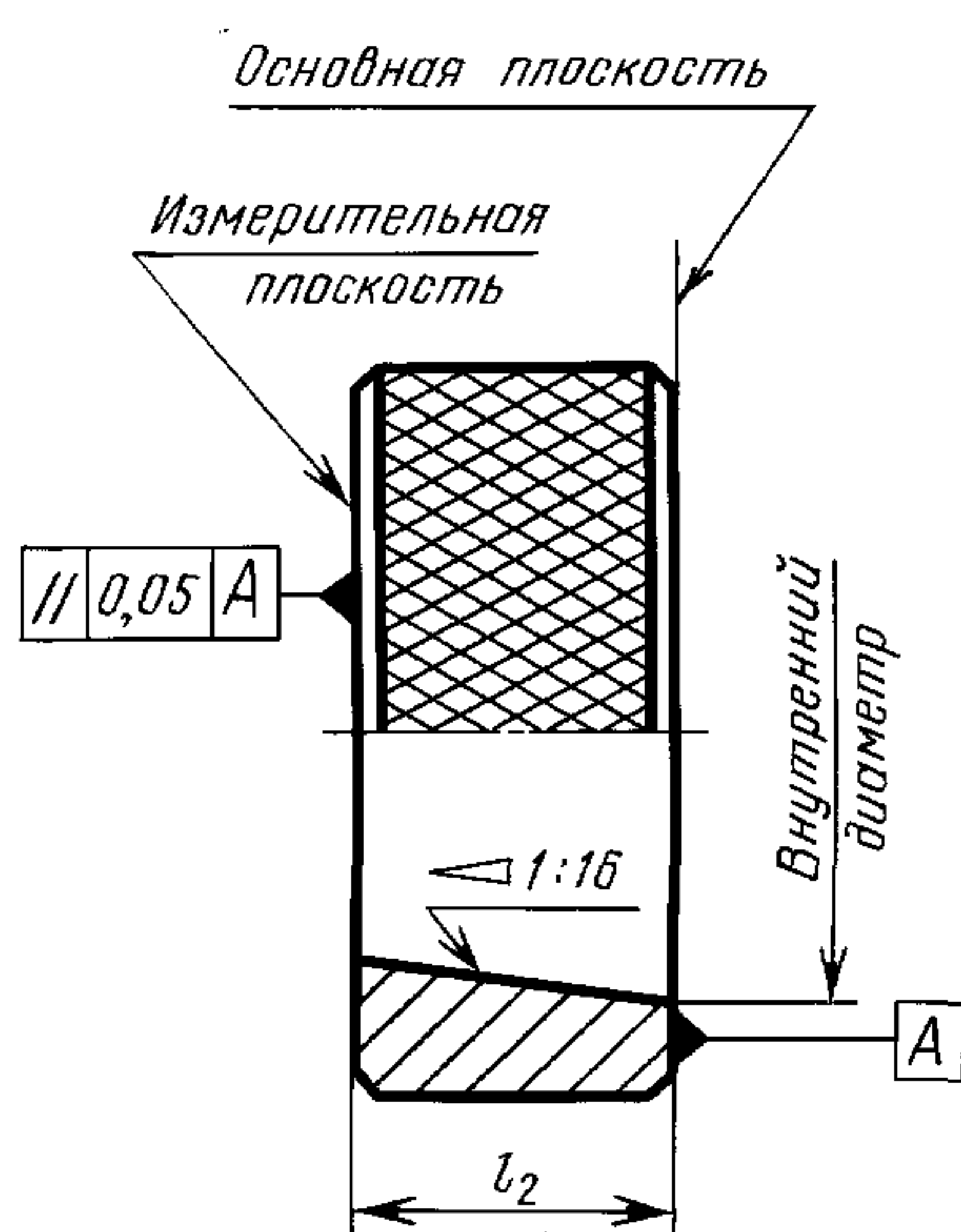
Калибр-кольцо Г
