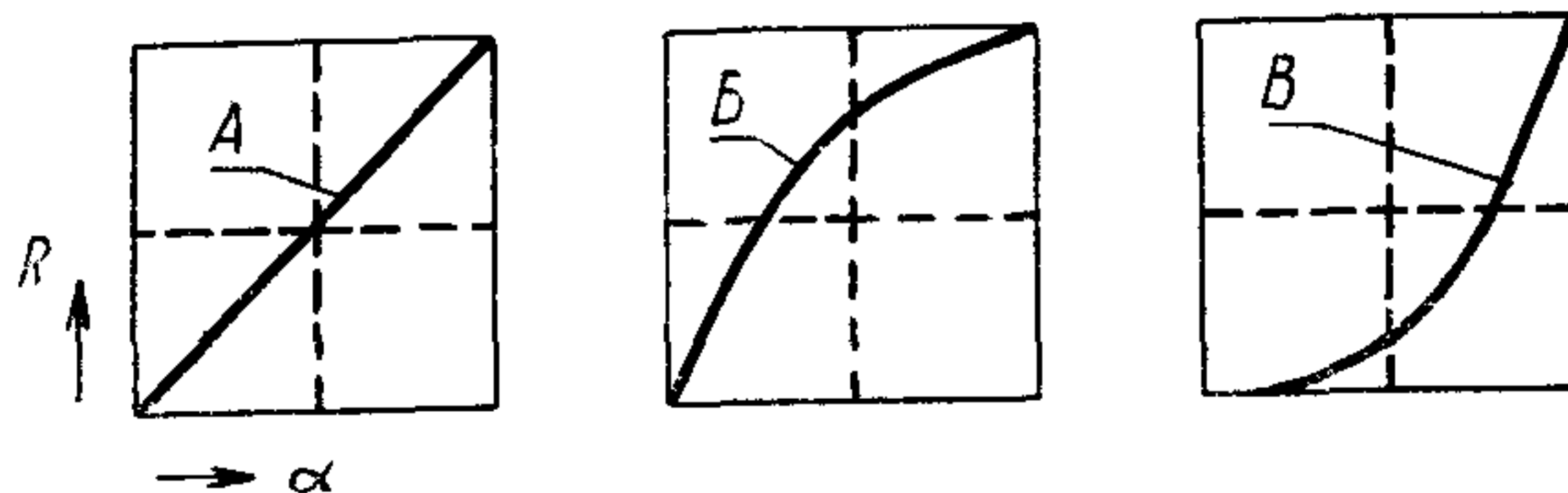
R —сопротивление; \alpha —рабочий угол поворота подвижной системы резистора; А—линейная зависимость; Б—нелинейная обратнoлогарифмическая зависимость; В—нелинейная лoгарифмическая зависимость
